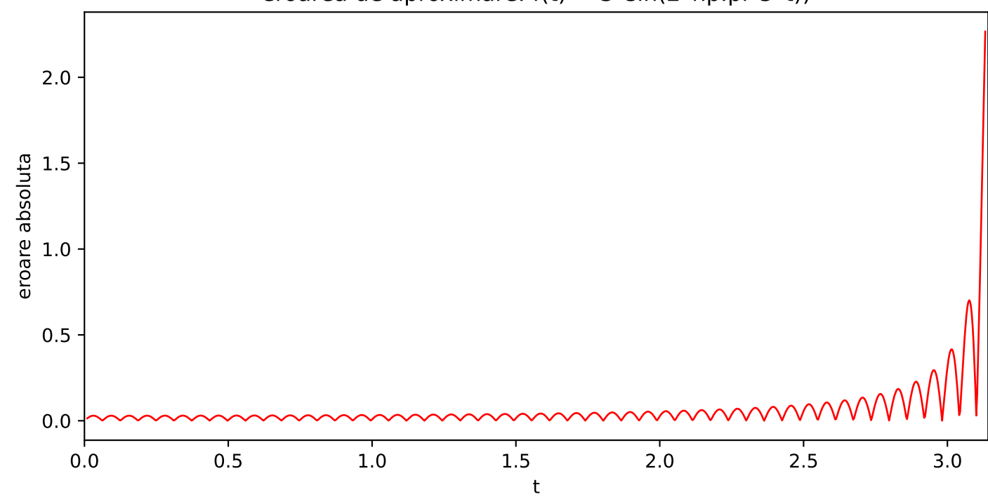
eroarea de aproximare: f(t) = 3 \sin(2\pi \cdot 5 \cdot t)
