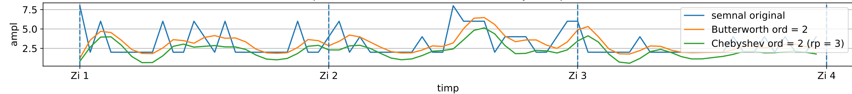
comparare semnale Butterworth si Chebyshev pe 3 zile
