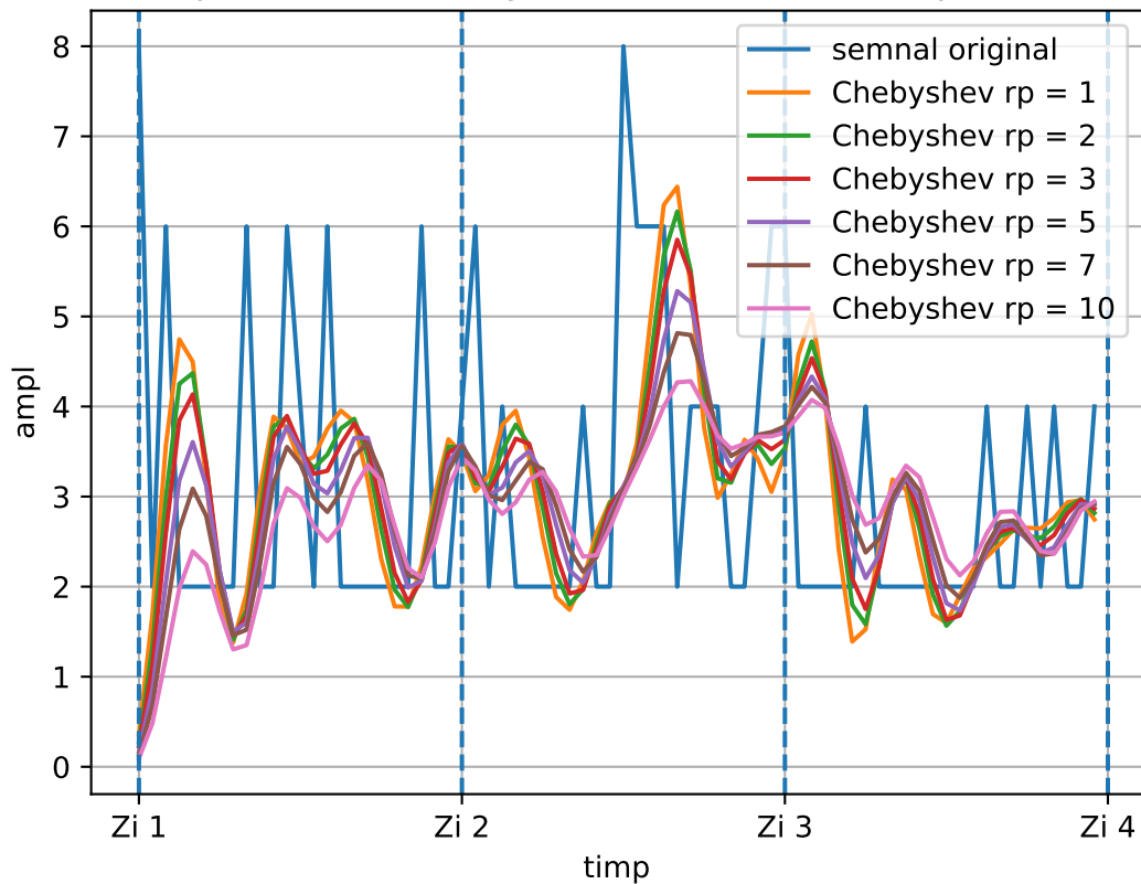
comparare filtre Chebyshev cu diferite valori r_p , ord = 3
