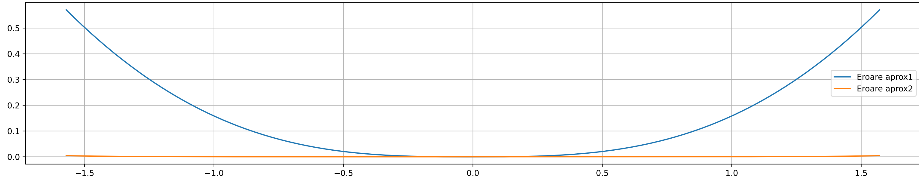
Eroare logaritmica
