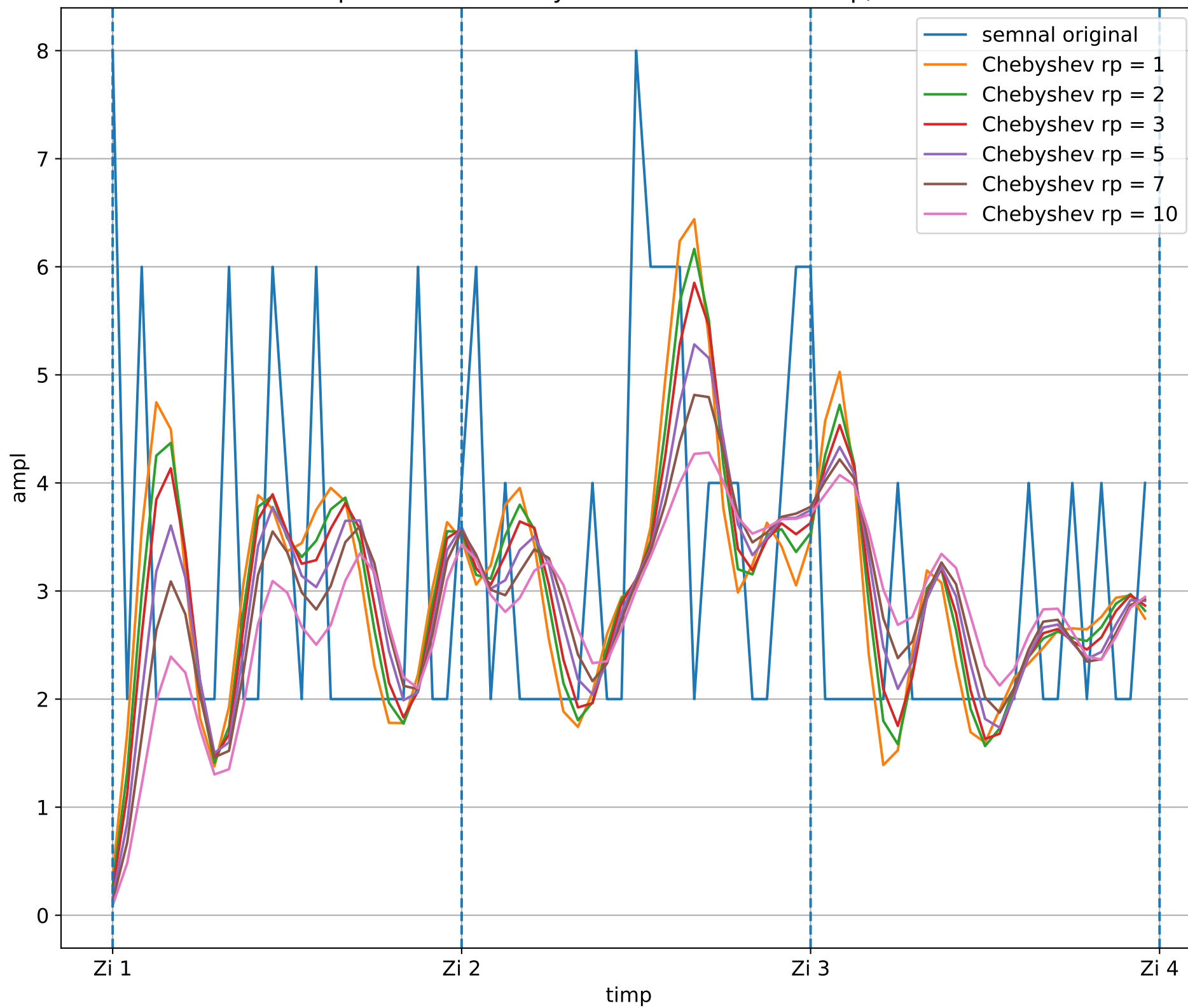
comparare filtre Chebyshev cu diferite valori rp, ord = 3
