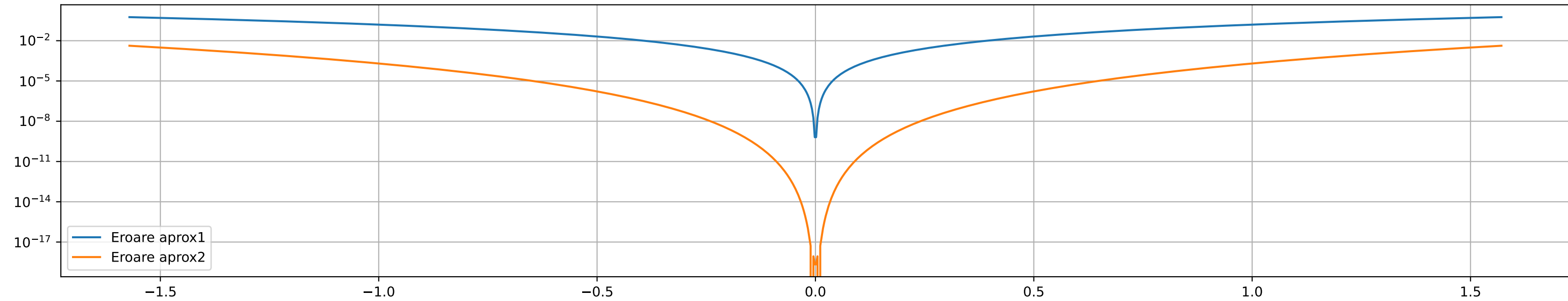
Eroare logaritmica
