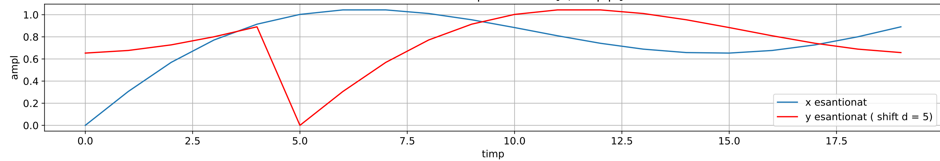
semnal esantionat cu 3 perioade pe intervalele: [0.0, 6.3] , [6.3, 12.6] , [12.6, 18.8]
