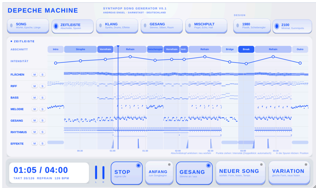
Abbildung 4: Die Zeitleiste eines Songs von vier Minuten: oben die Abschnitte, darunter die Intensitätskurve und die Noten der sieben Spuren; die senkrechte Linie ist die Abspielposition im ersten Refrain
