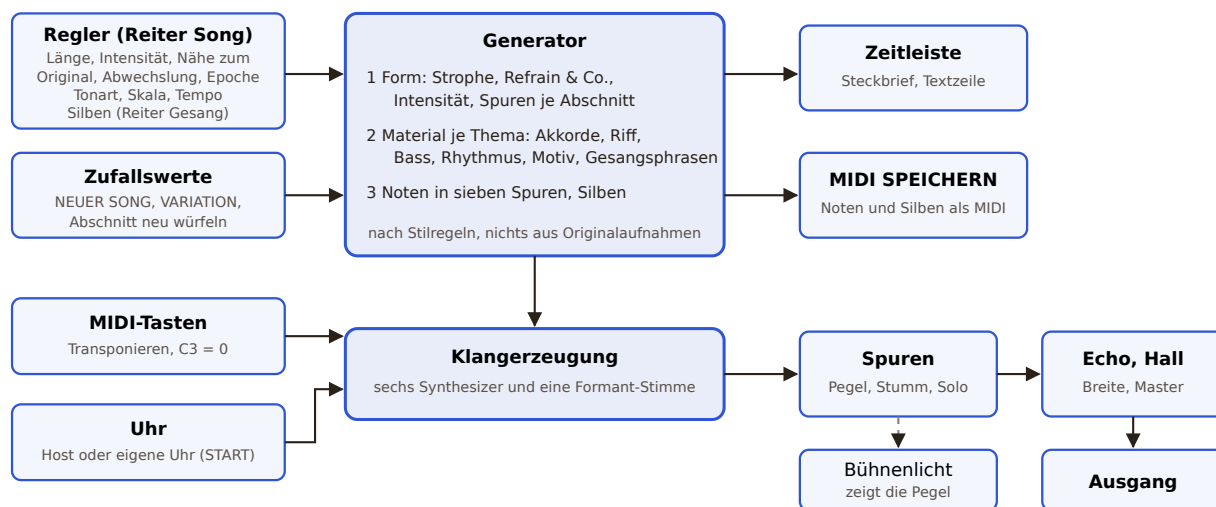
Abbildung 2: Vom Würfel zum Klang: so entsteht ein Song in DEPECHE MACHINE
