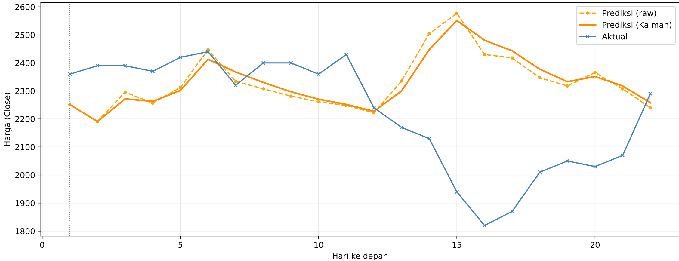
AMRT — Prediksi 22 Hari ke Depan (dari 2025-02-28)
