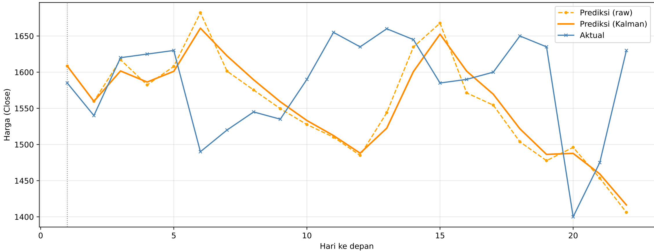
ANTM — Prediksi 22 Hari ke Depan (dari 2025-02-28)
