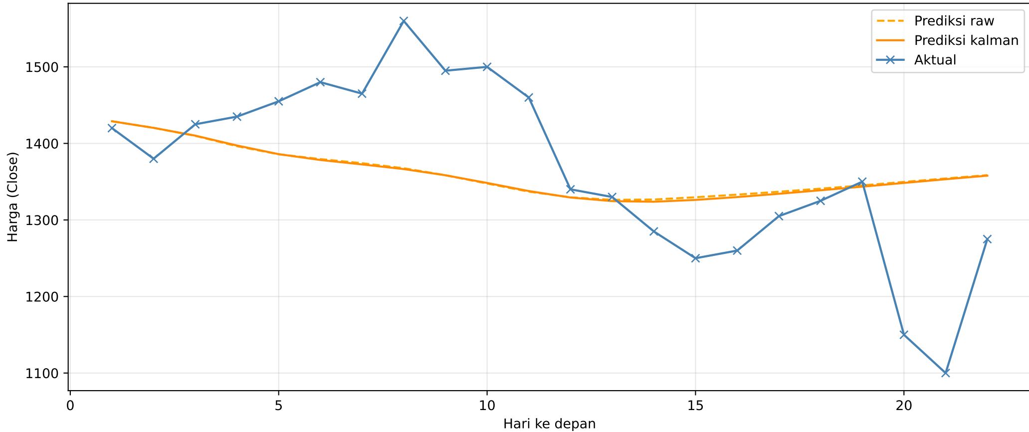
MAPI - Prediksi 22 Hari
