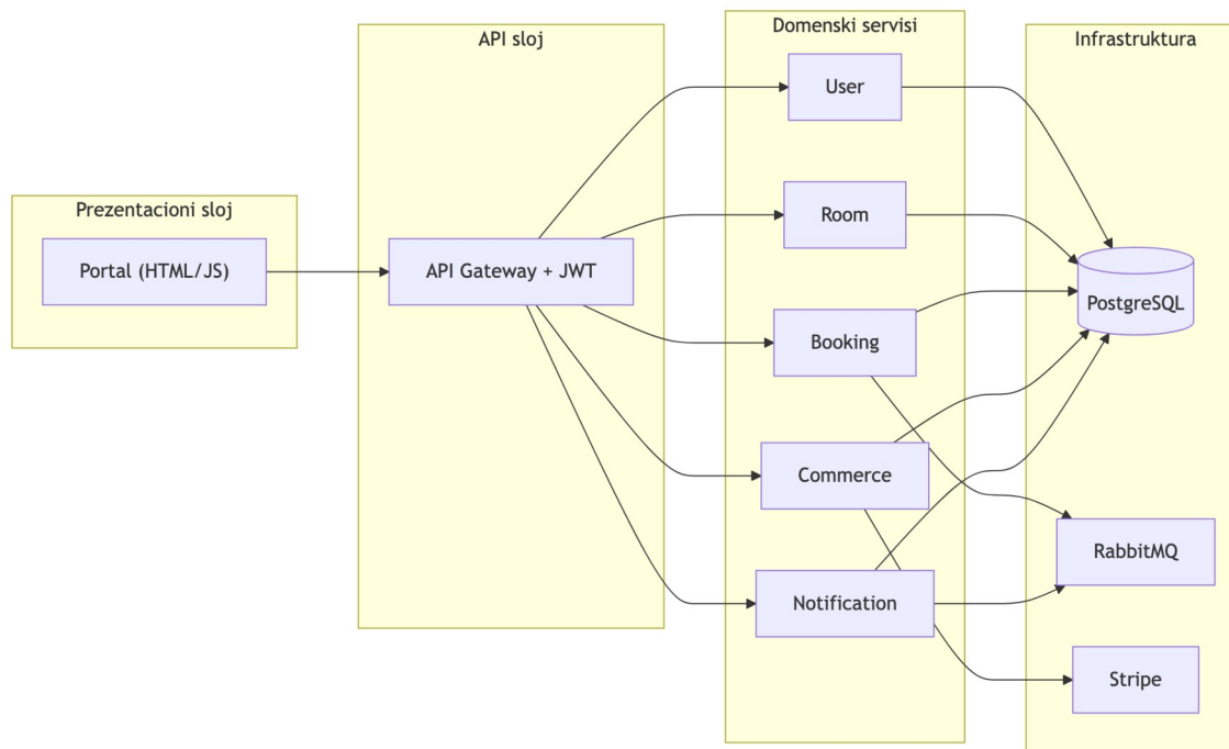
Slika 3. Arhitektura aplikacije
