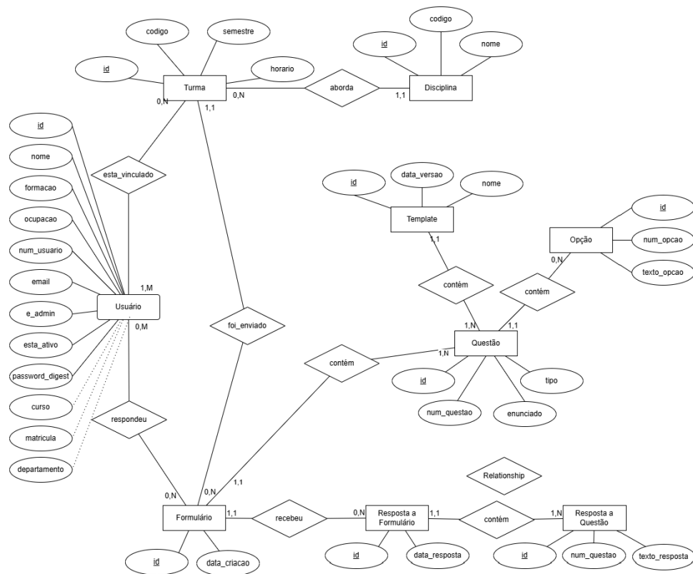
Figure 1: Modelo Entidade-Relacionamento conceitual.
