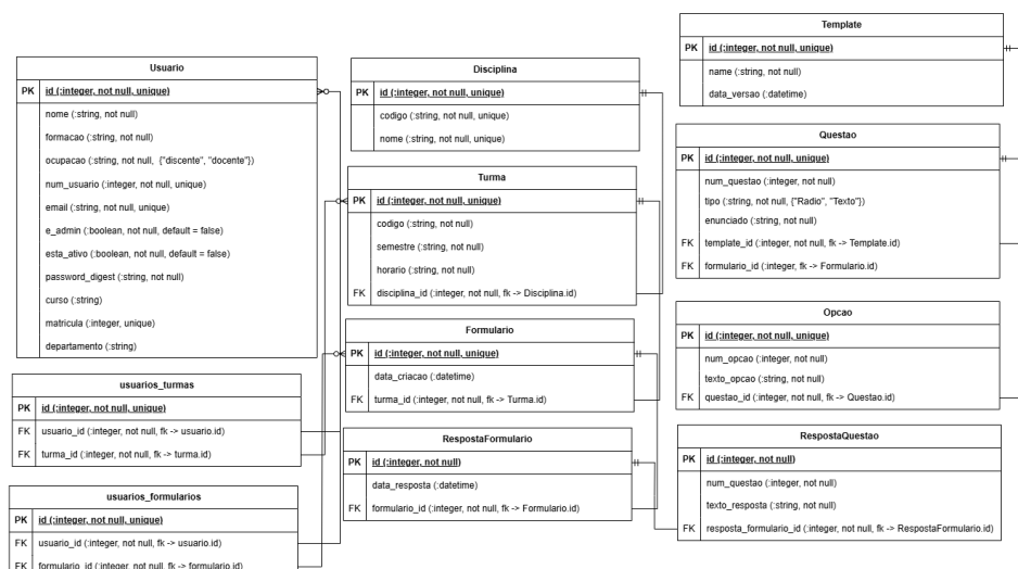
Figure 2: Modelo Entidade-Relacionamento lógico.
