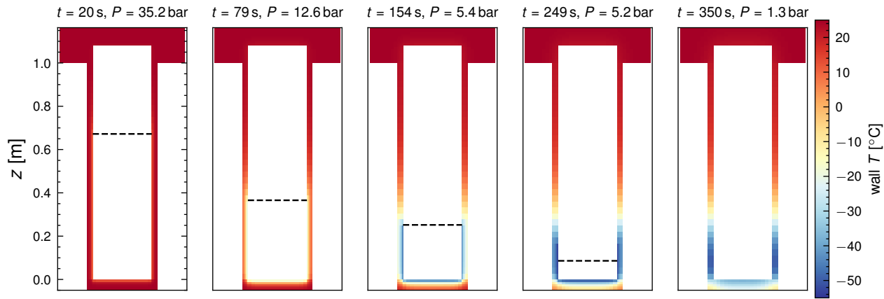
Exp72 (no-riser / gas)
