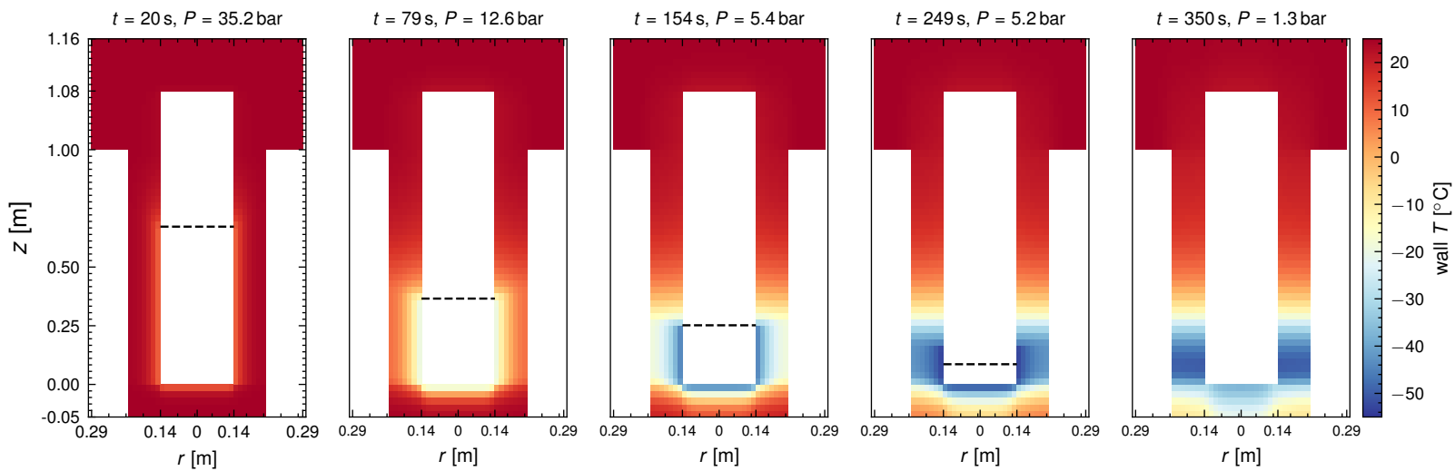
Exp72 (no-riser / gas)
