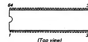
N50941-712SP
