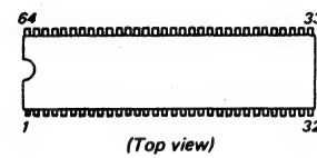
N50941-712SP
