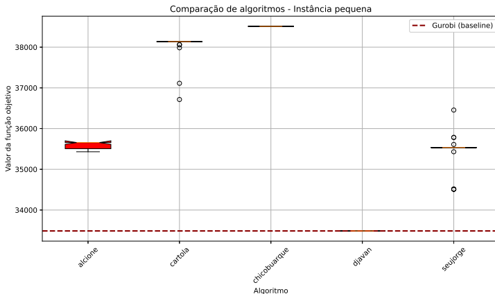
Figura: Boxplot dos resultados para a instância pequena.
