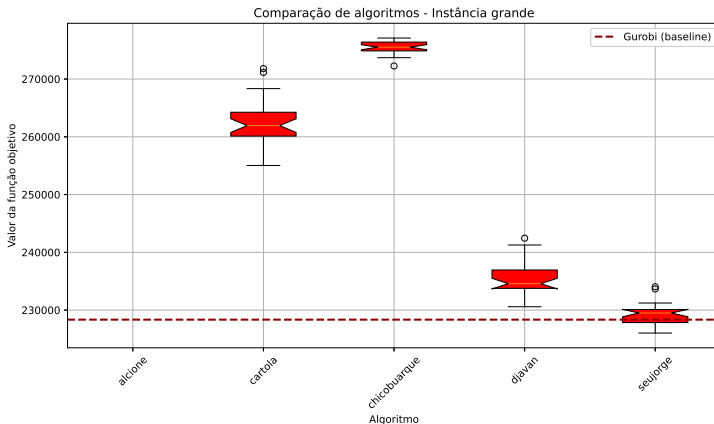
Figura: Boxplot dos resultados para a instância grande.
