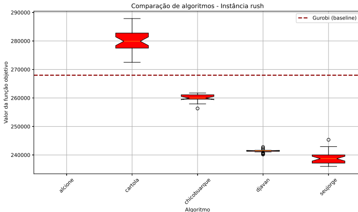
Figura: Boxplot dos resultados para a instância rush.
