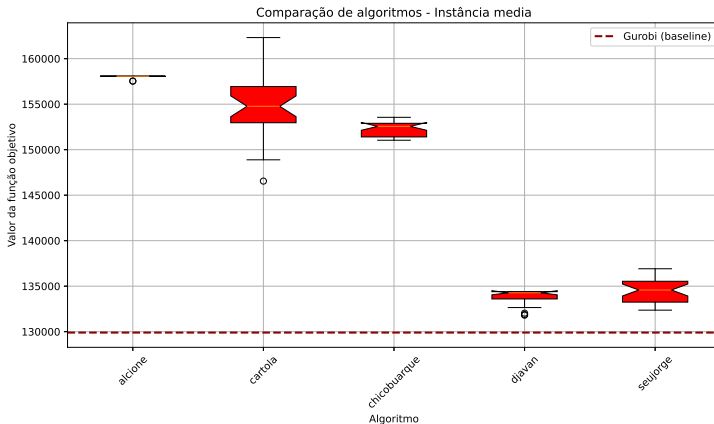
Figura: Boxplot dos resultados para a instância média.
