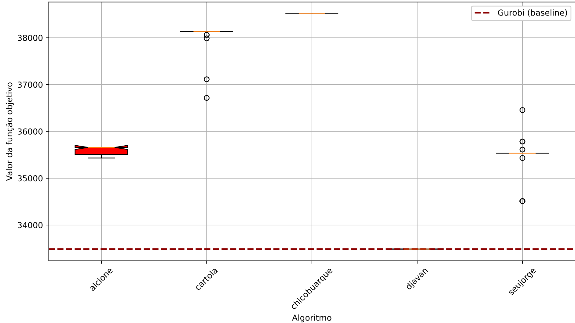
Comparação de algoritmos - Instância pequena
