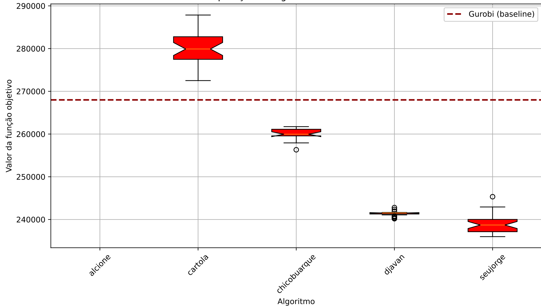
Comparação de algoritmos - Instância rush
