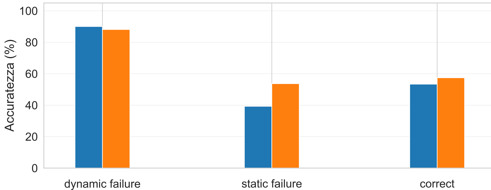
Valutazione Output
