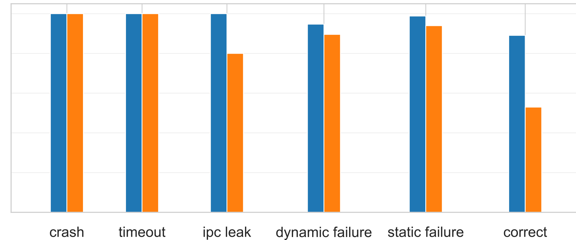
Valutazione Codice
