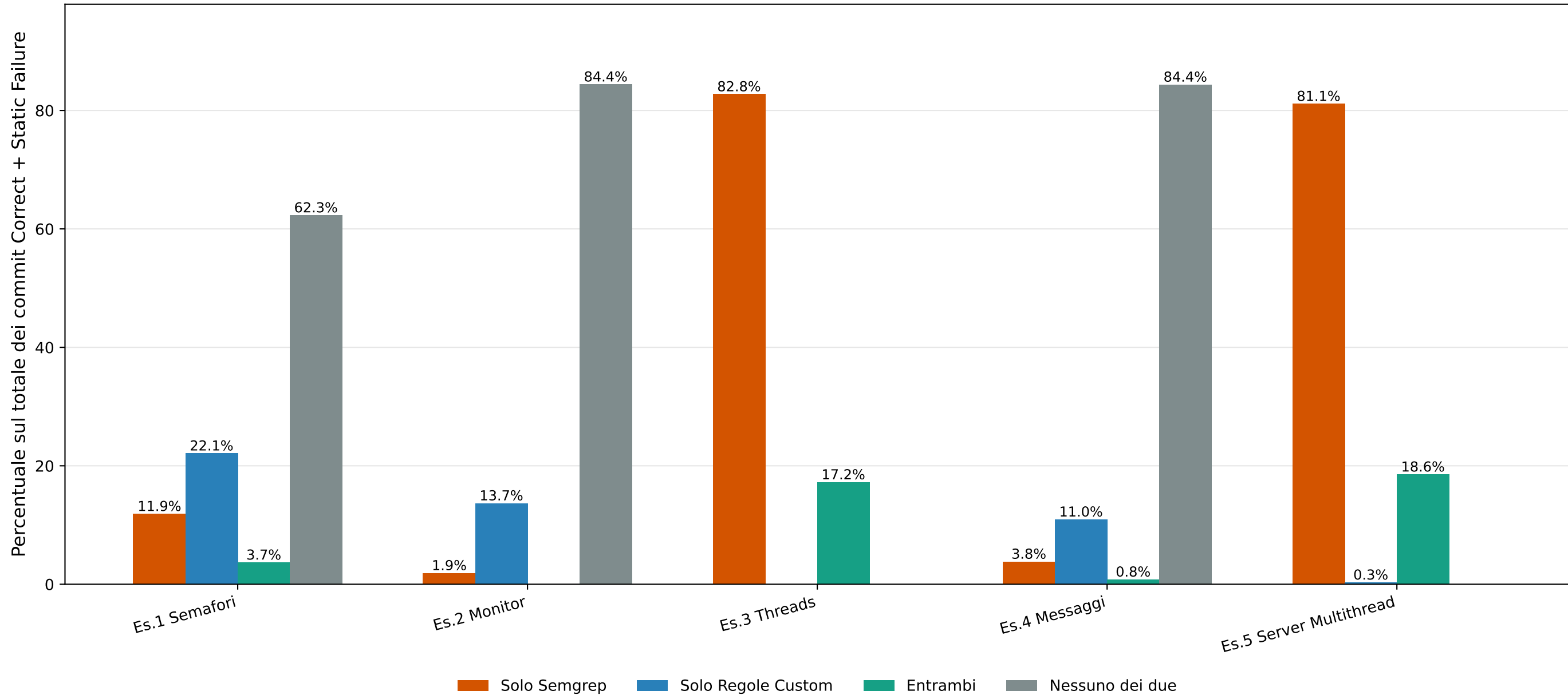
Sovrapposizione tra Semgrep e Regole Custom su commit Correct + Static Failure
