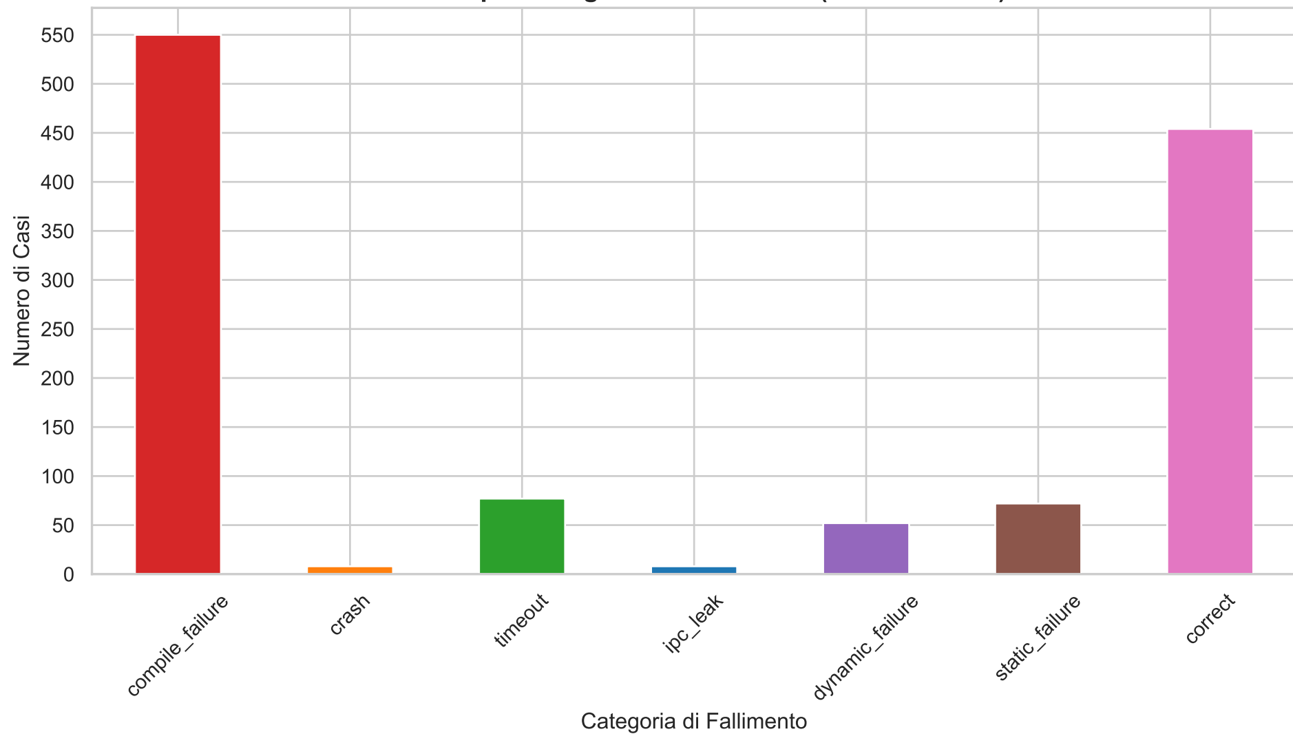
Distribuzione dei Casi per Categoria di Fallimento (Tutti i Commit) - Es.2 Monitor
