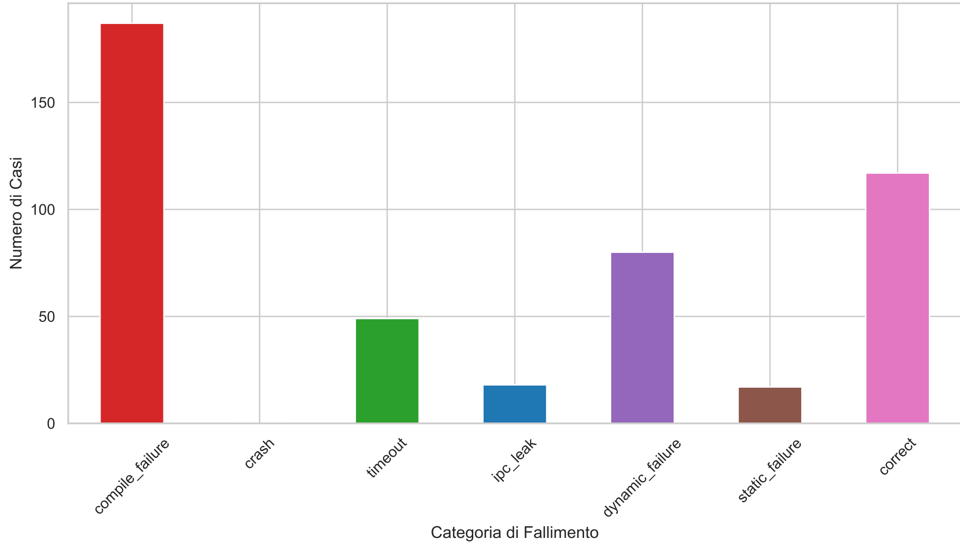
Distribuzione dei Casi per Categoria di Fallimento - Es.4 Messaggi
