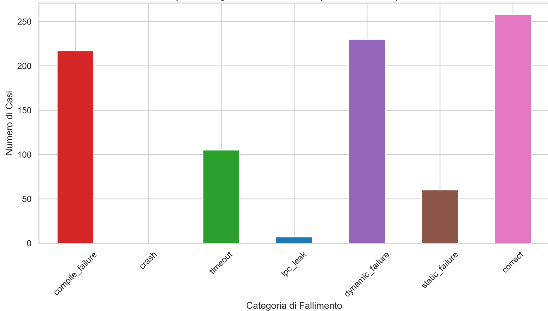
Distribuzione dei Casi per Categoria di Fallimento (Tutti i Commit) - Es.5 Server Multithread
