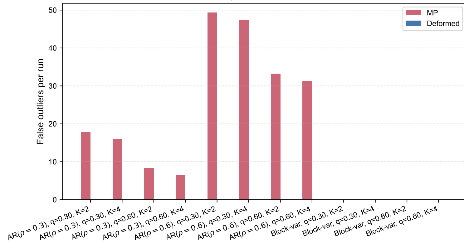
9B) False outlier rate
