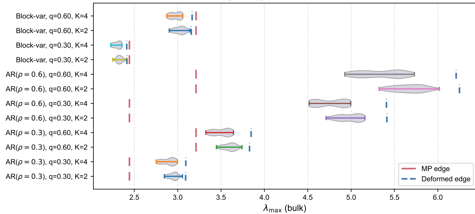
9A) Bulk spectrum vs thresholds
