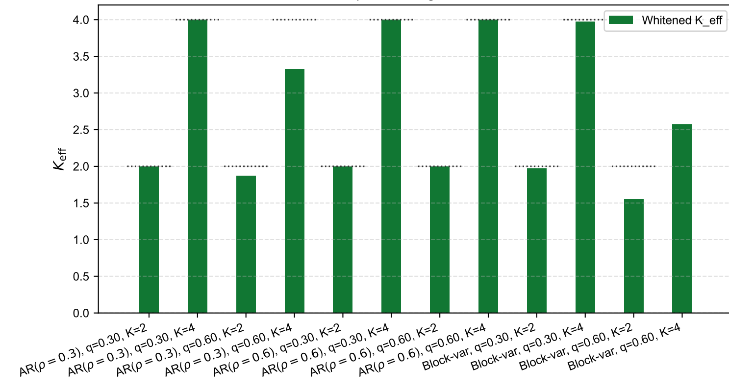
9D) Whitening ablation
