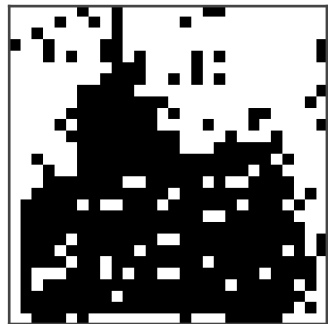
Noisy Input
