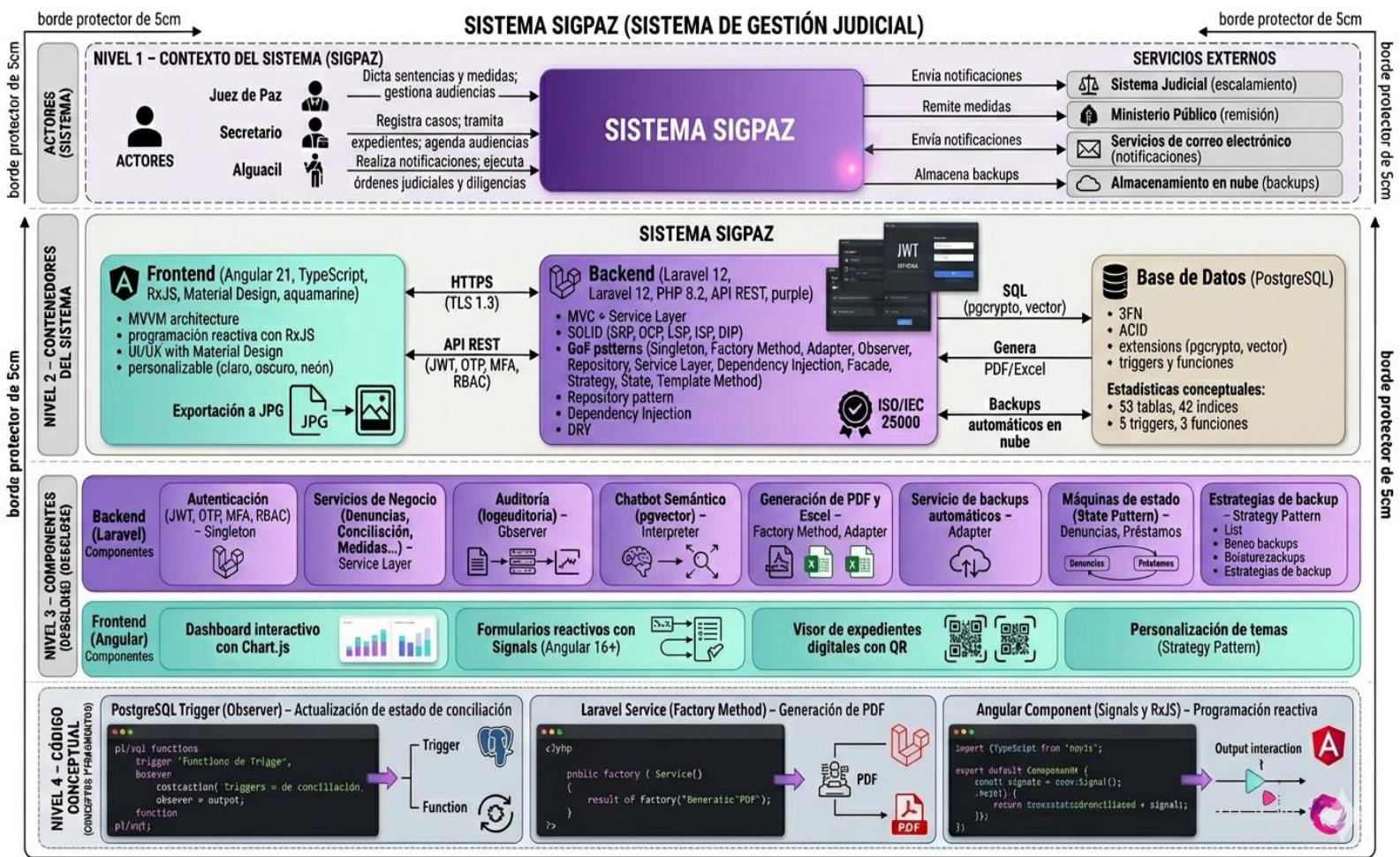
12) FIGURA: DIAGRAMA DEC4 DE SISTEMA PROPUESTO
