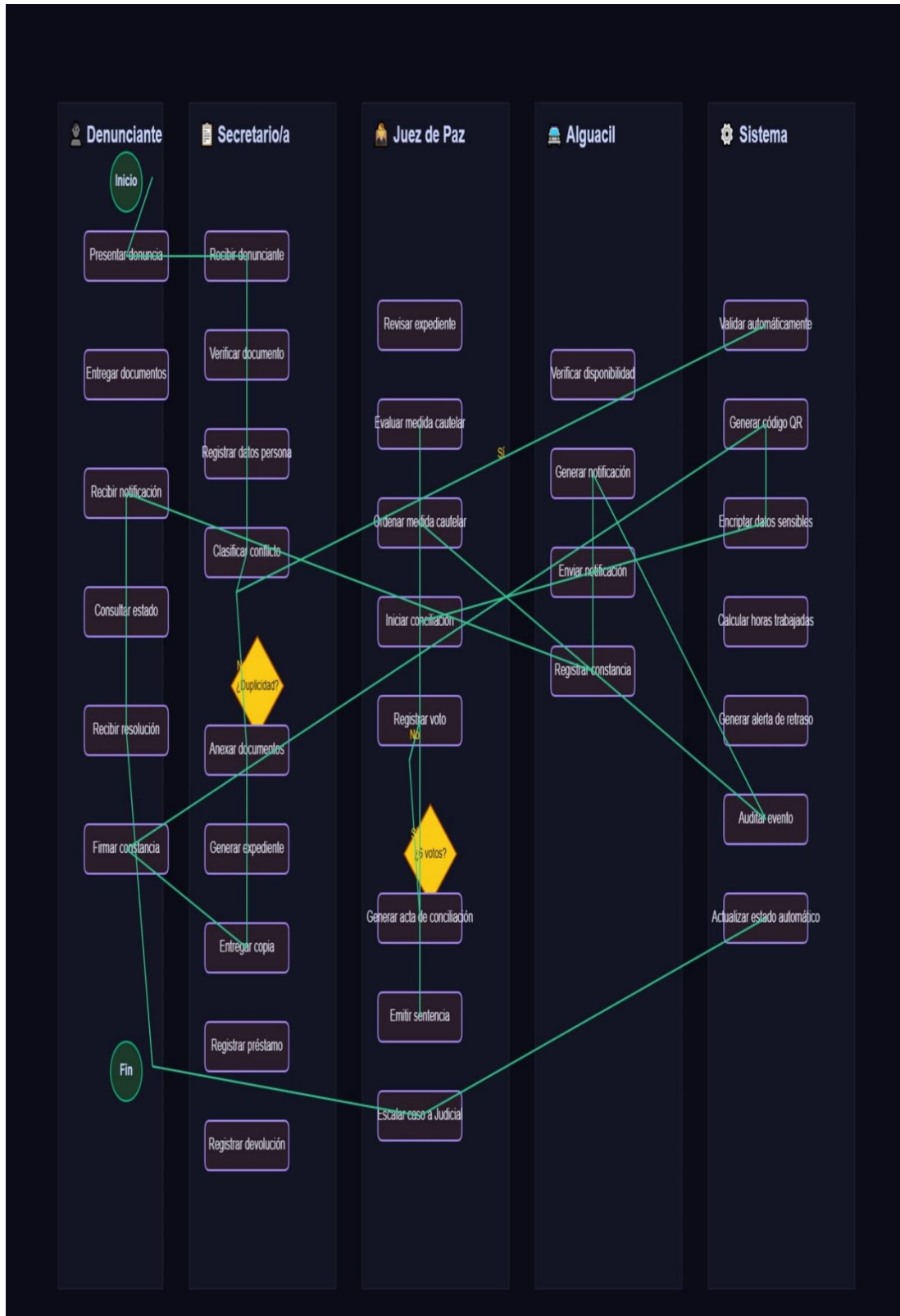
20) FIGURA: DIAGRAMA DE ACTIVIDADES (PROPUESTO)
