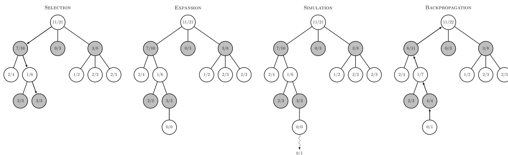
Figura 2: I 4 step della ricerca ad albero di Monte Carlo
