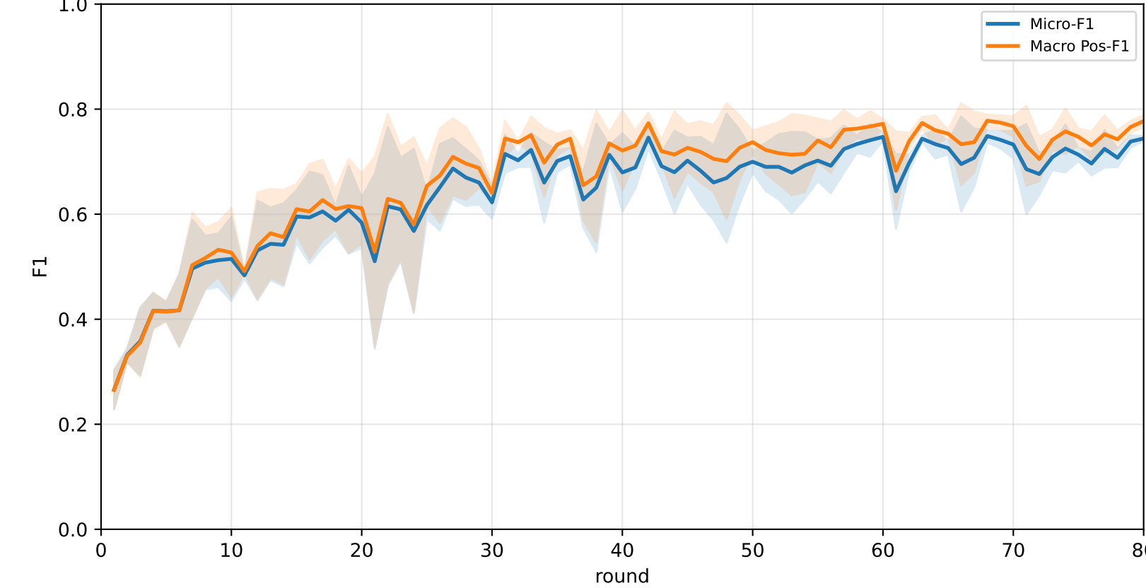
Pooled Local baseline micro / macro F1
