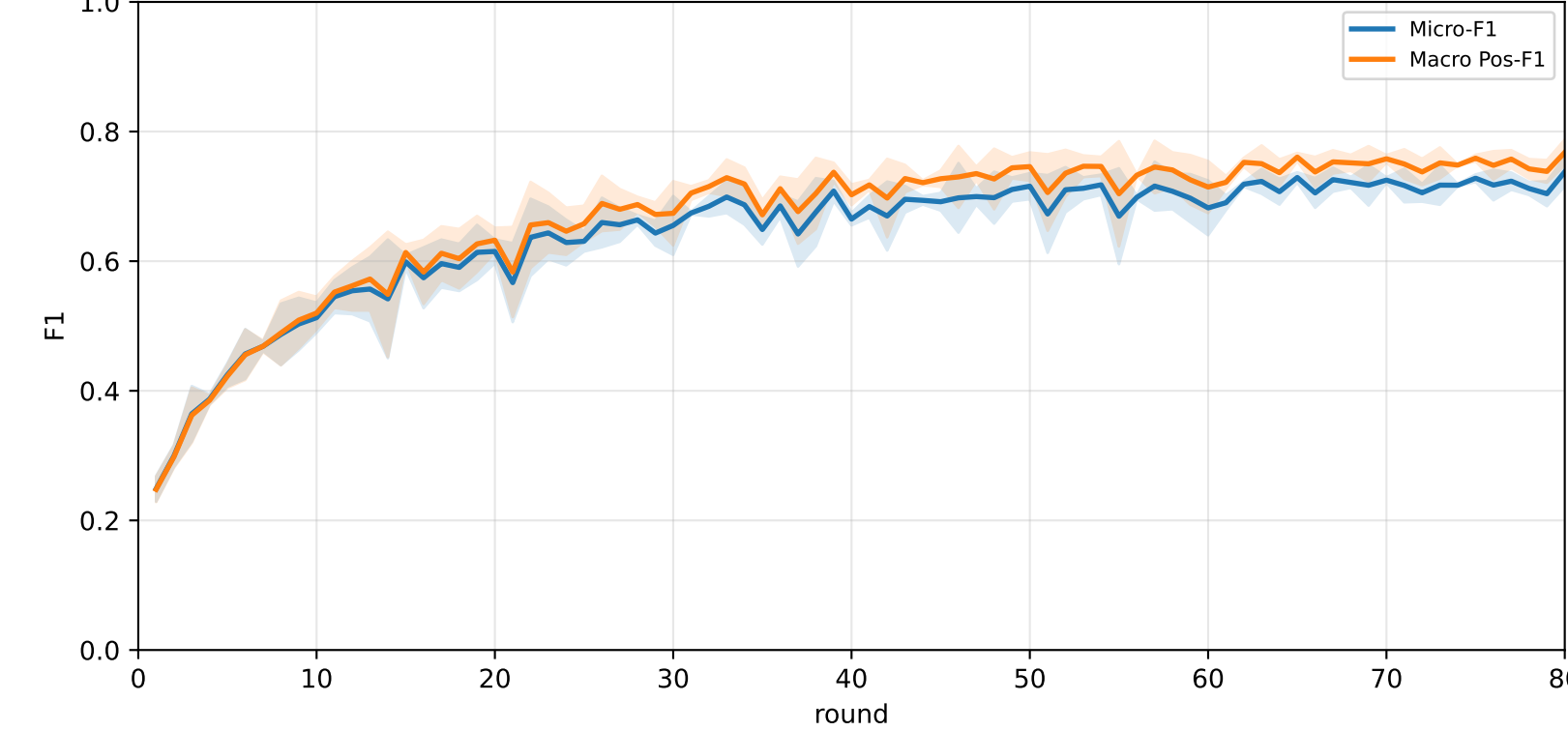
Pooled Local baseline micro / macro F1
