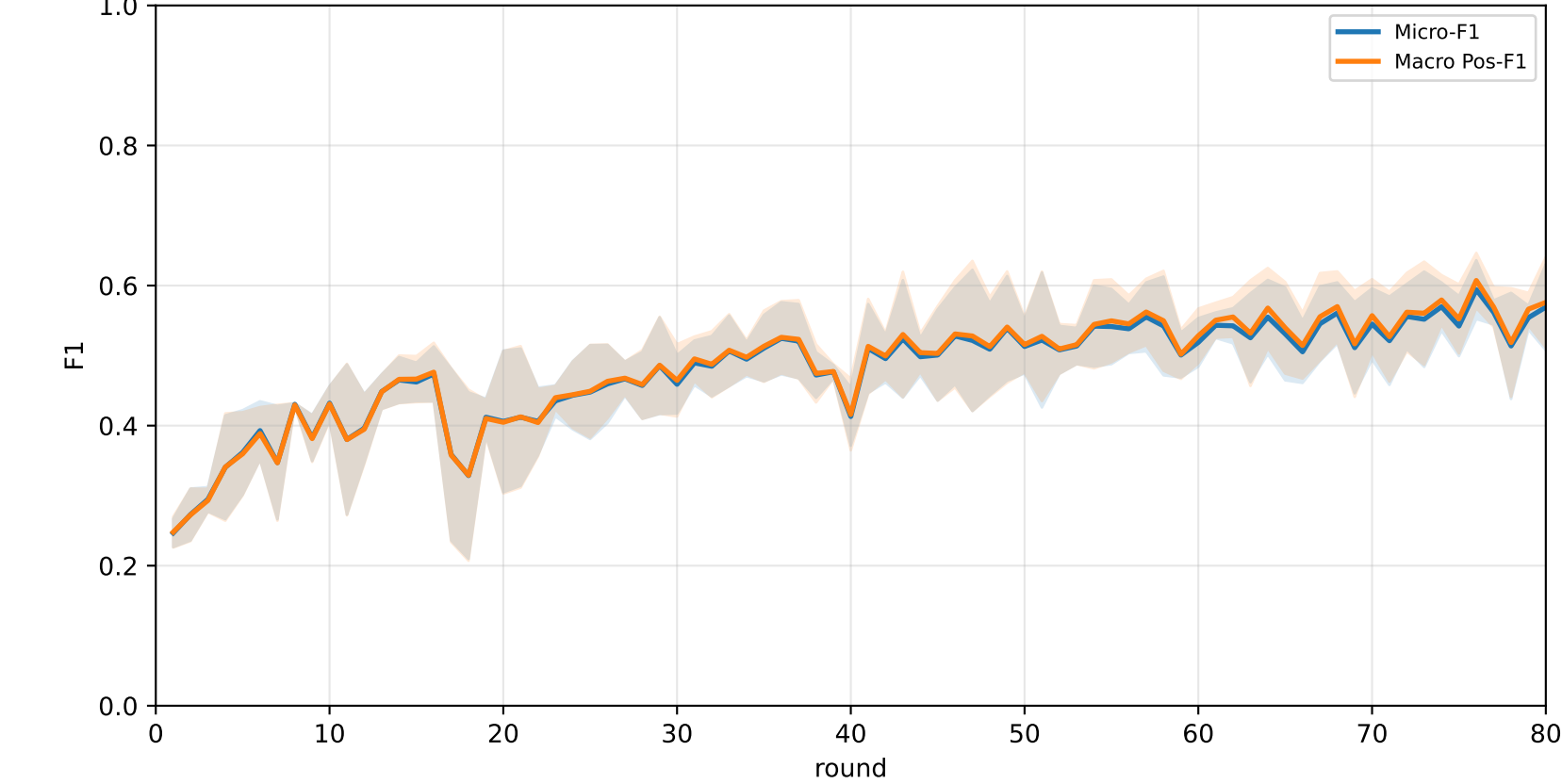
Pooled Local baseline micro / macro F1
