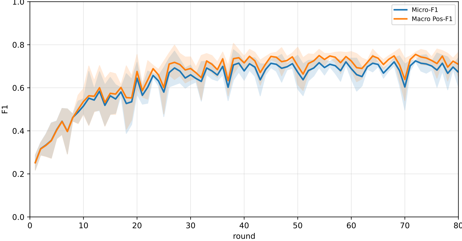
Pooled Local baseline micro / macro F1
