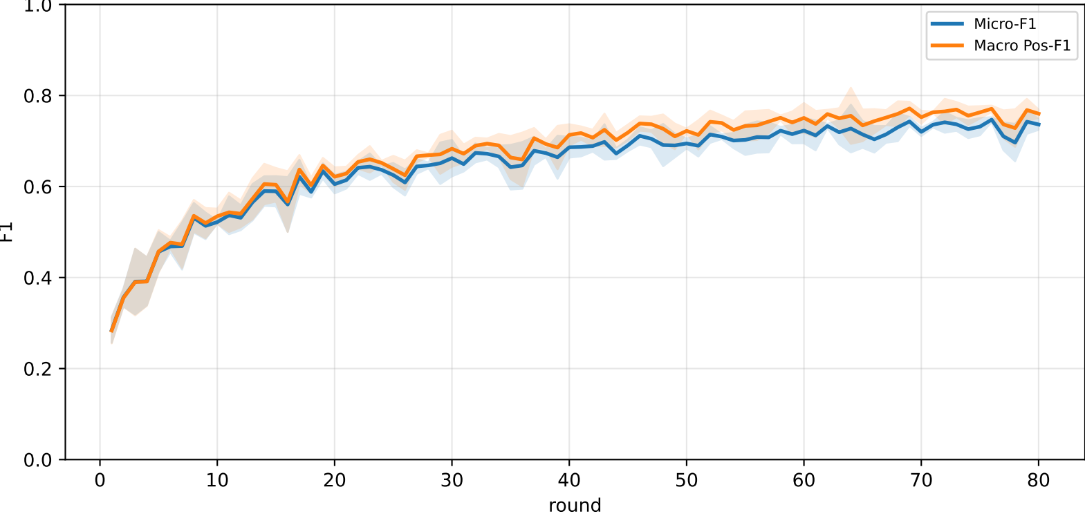
Pooled local centralized micro / macro F1
