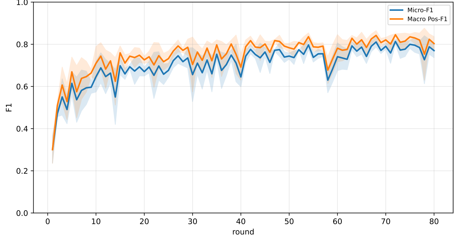
Pooled local centralized micro / macro F1
