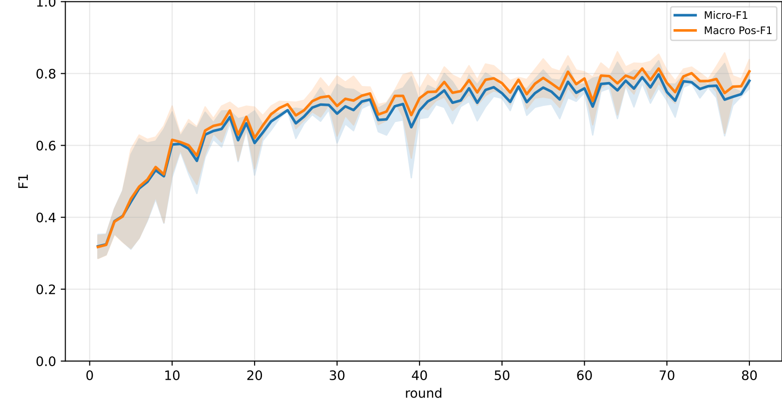
Pooled local centralized micro / macro F1
