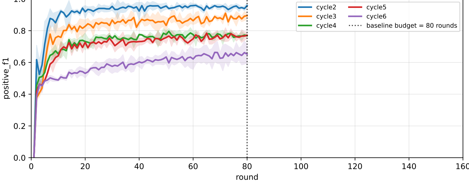
Pooled GCFL+ positive F1
