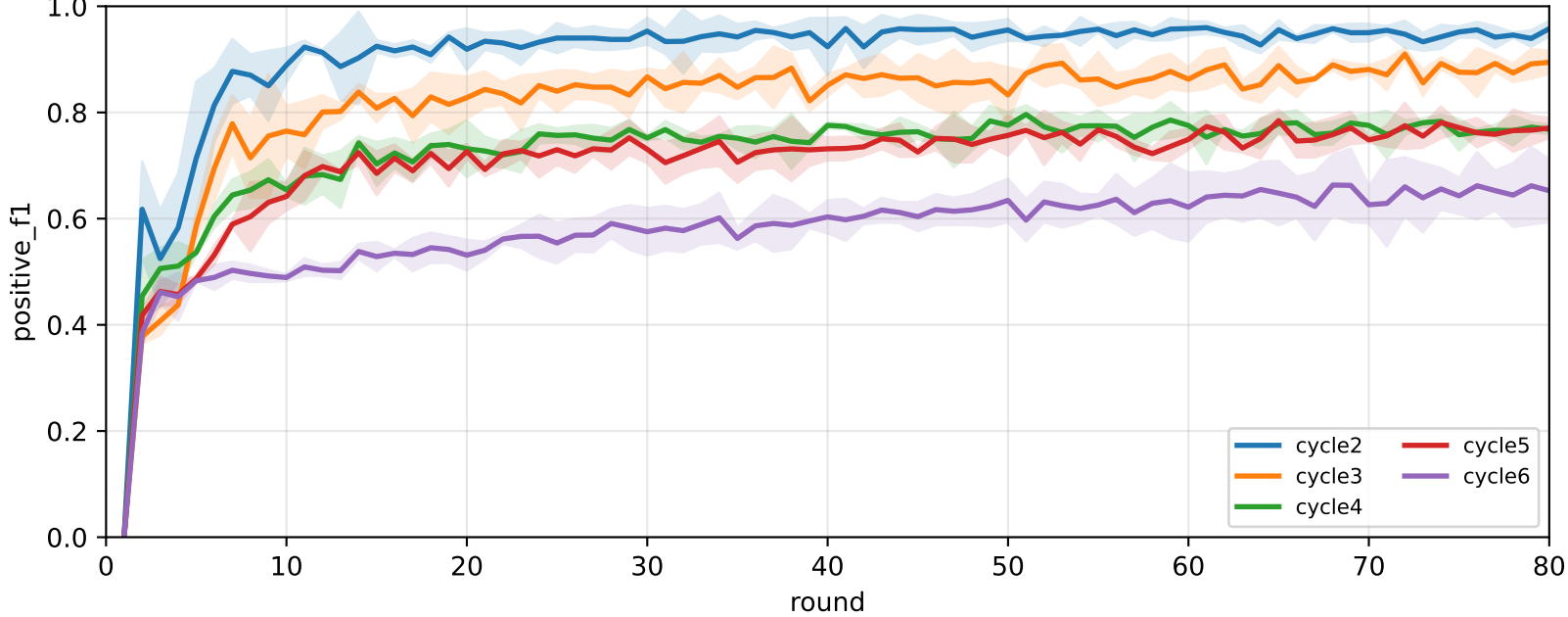
Pooled FedAvg positive F1
