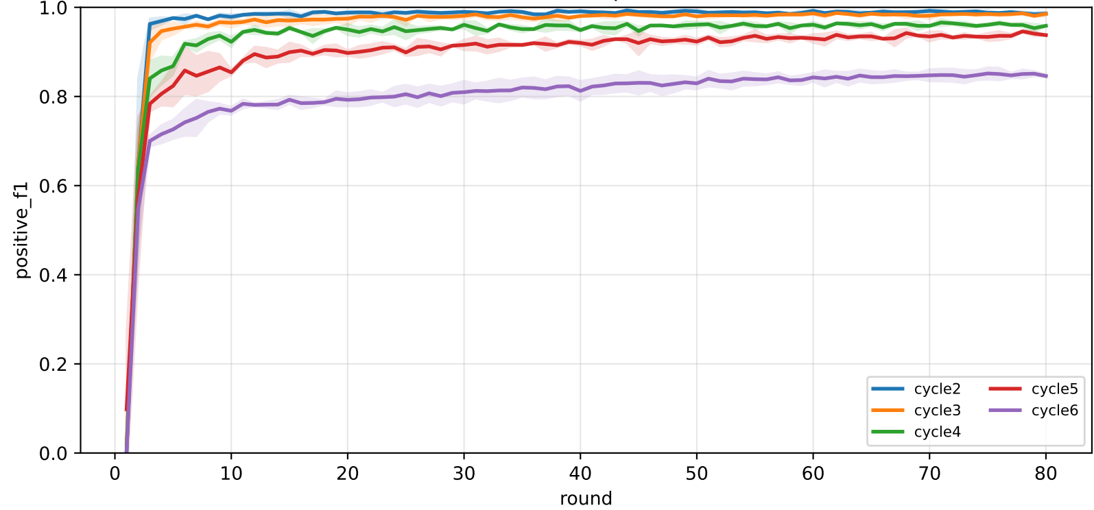
Pooled FedProx positive F1
