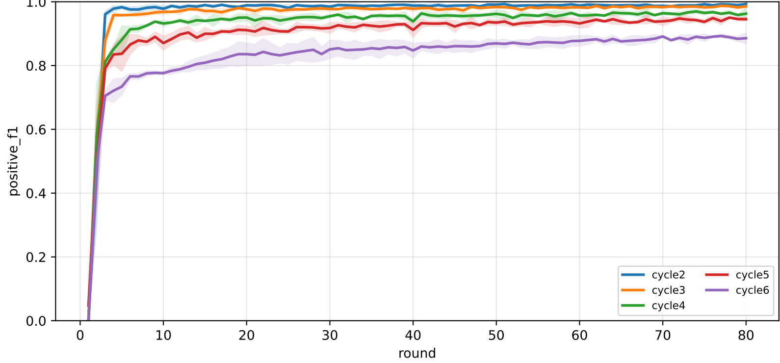
Pooled FedAvg positive F1
