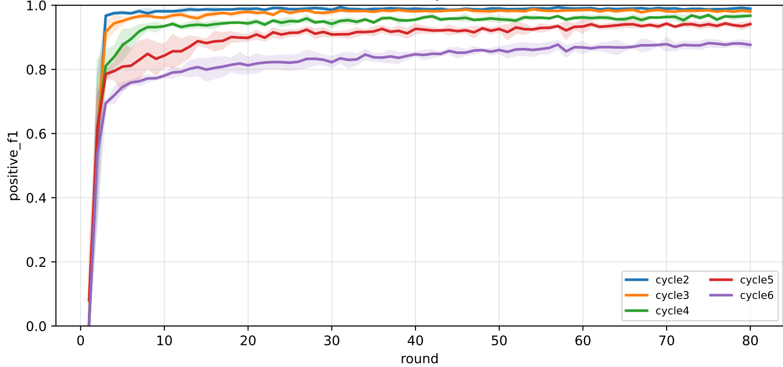
Pooled GCFL+ positive F1
