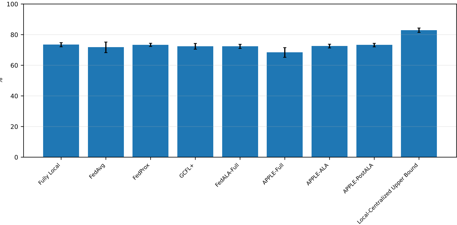
Micro PR-AUC
