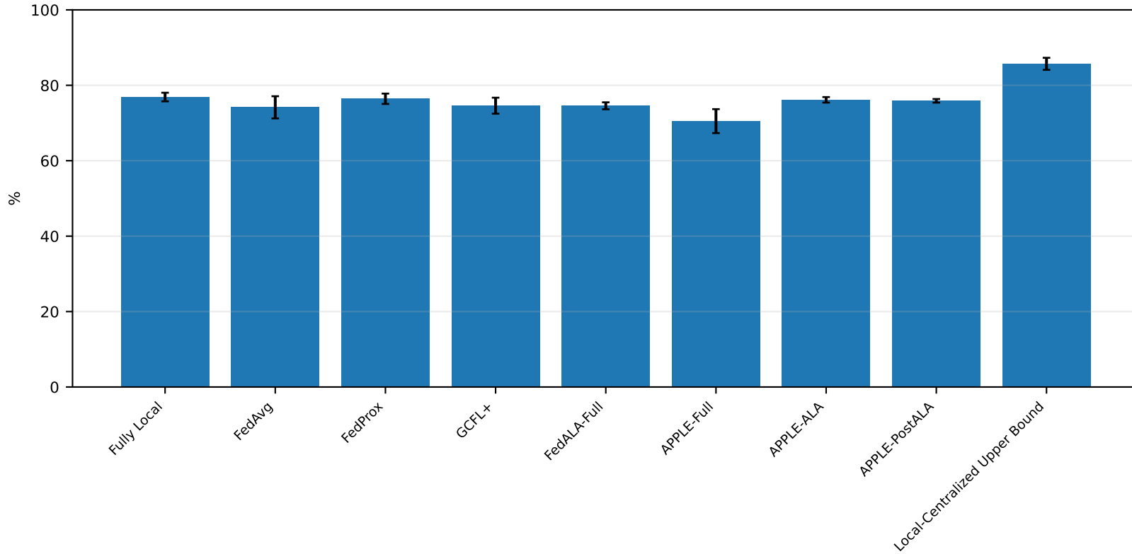
Macro PR-AUC
