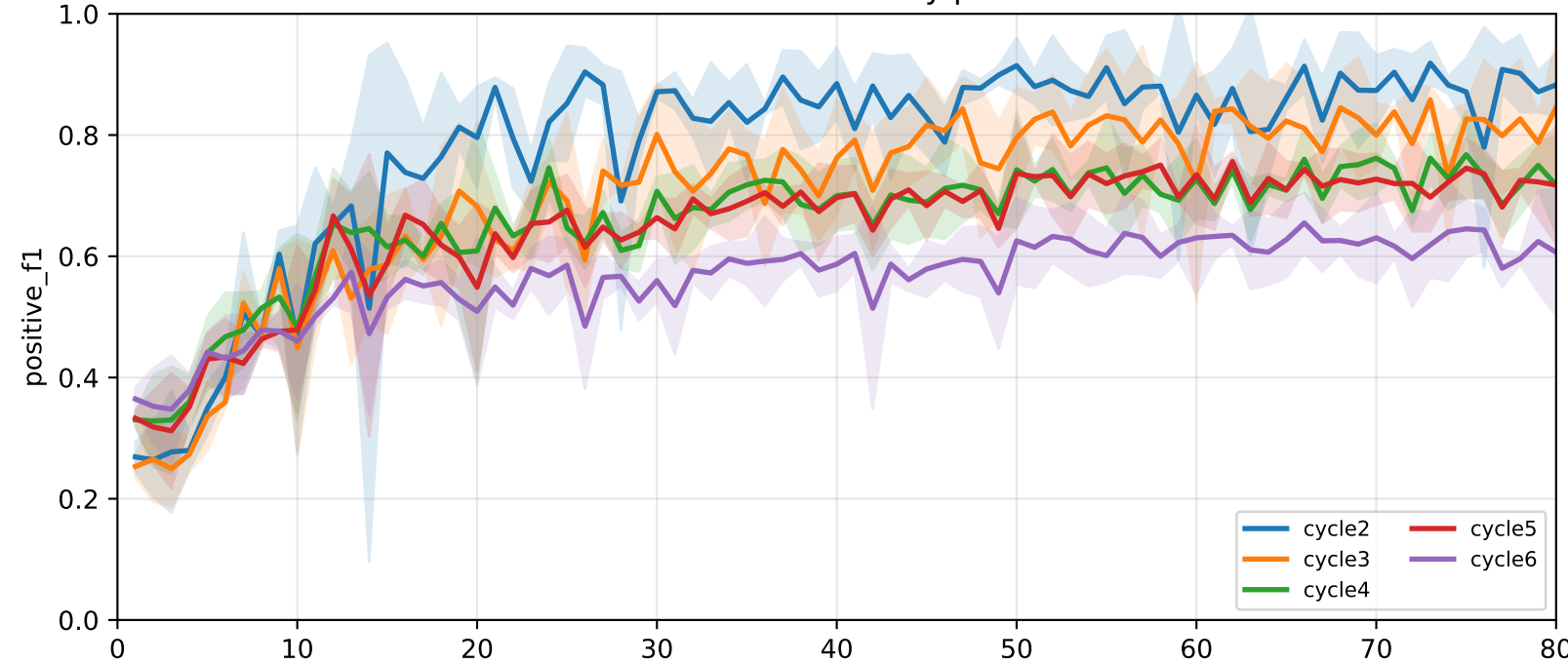
Pooled FedALA-HeadOnly positive F1
