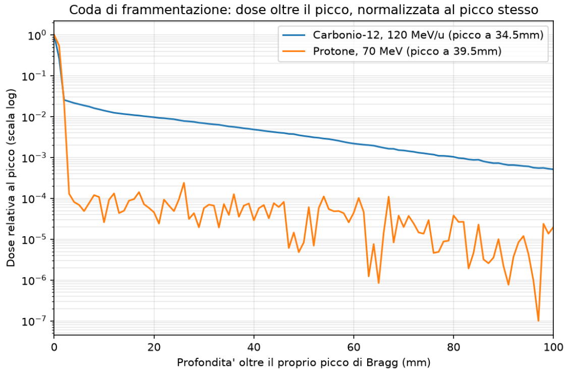
Fig. 53 — Coda di frammentazione oltre il picco di Bragg: dose relativa al picco (scala log) in funzione della profondita' oltre il proprio picco, carbonio-12 120 MeV/u contro protone 70 MeV. Il carbonio mostra una coda liscia e persistente; il protone crolla quasi subito a un livello rumoroso \sim 300\times piu' basso.
