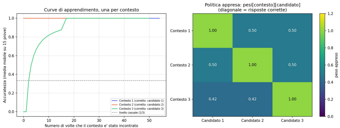
Fig. 18 — Curve di apprendimento per contesto (sinistra); politica finale appresa, tabella pesi[contesto][candidato] (destra).
