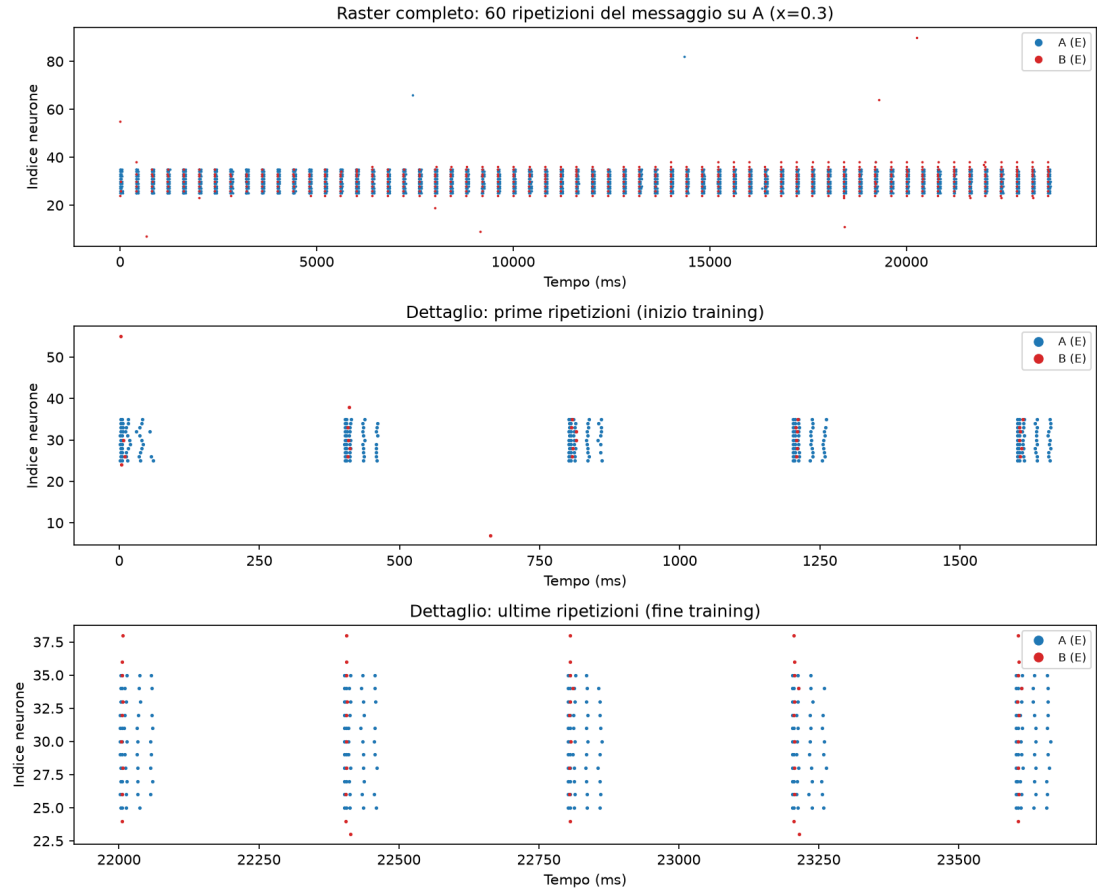
Fig. 35 — Tentativo di bidirezionalita' spiking: A->B continua a funzionare, B->A non mostra segnale di apprendimento in nessuna delle 60 ripetizioni.
