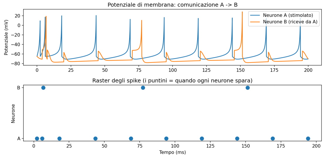
Fig. 1 — Potenziale di membrana e raster: comunicazione A \rightarrow B .
