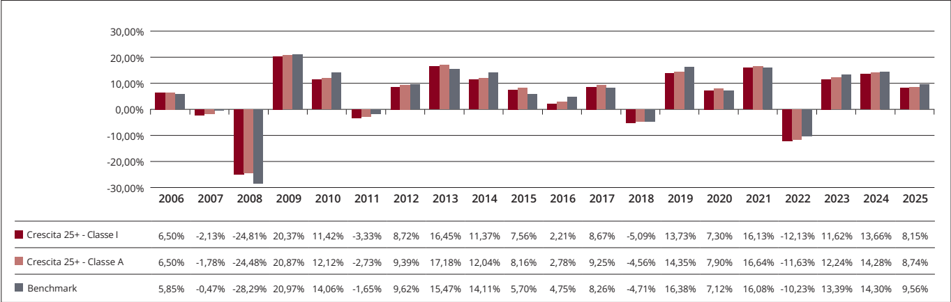
Rendimenti netti annui (valori percentuali) del Comparto Crescita 25+ e del benchmark
