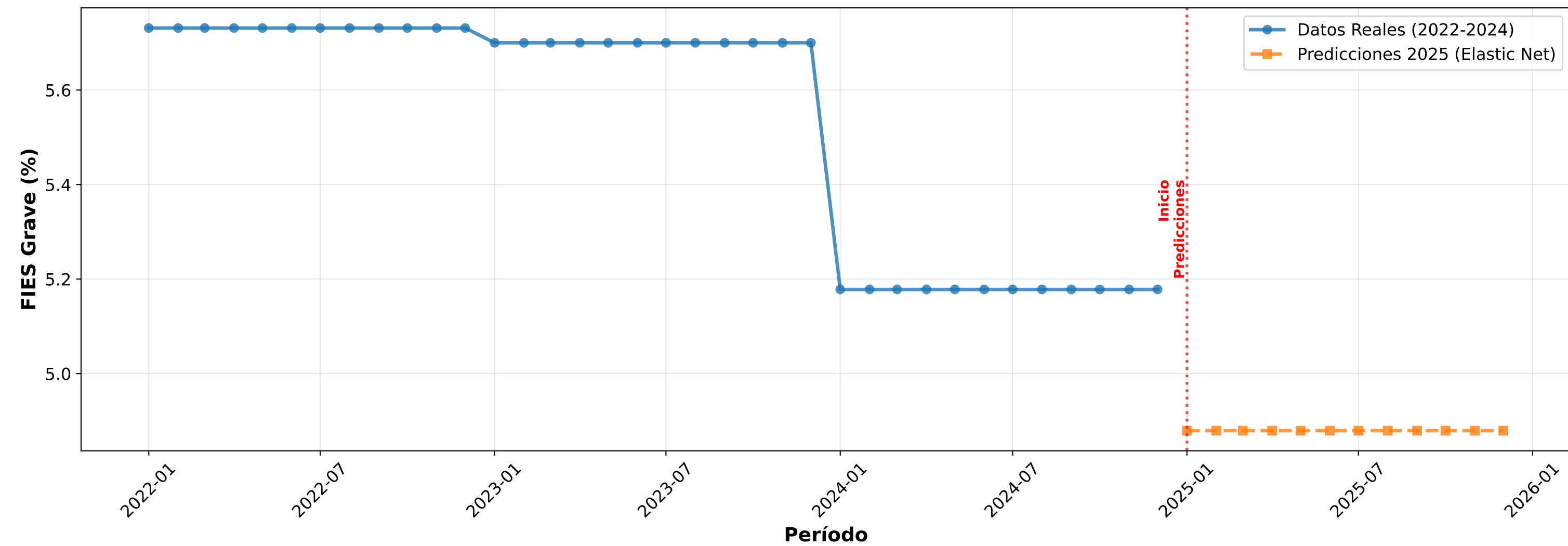
Evolución Temporal FIES Grave: Datos Reales vs Predicciones
