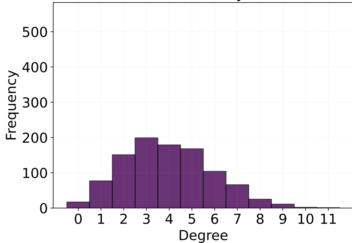
Erdős-Rényi
