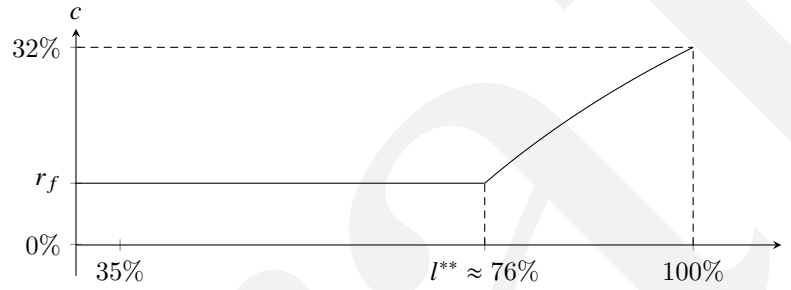
Fig. 6.5: Coupon c in Prob. 2.11.
