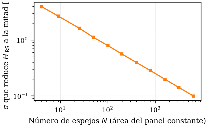
(b) Tolerancia al error de apuntamiento
