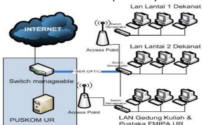
Gambar 1. Topologi Jaringan FMIPA Universitas Riau
