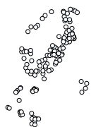
chr7_46281686_G_C E (n.d.)
