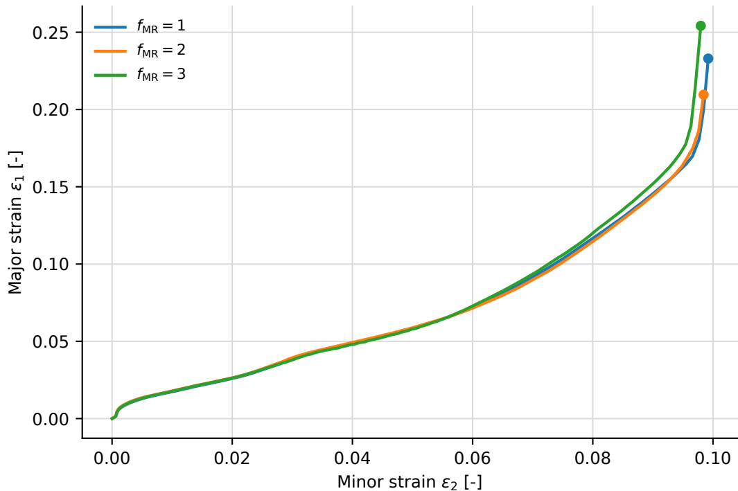
Mesh-refinement sensitivity ( \Delta t_{MS} = 10^{-5} s)
