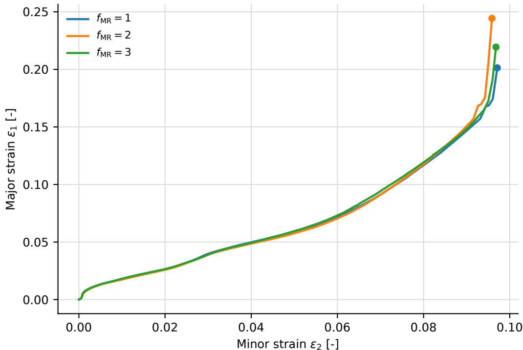
Mesh-refinement confirmation ( \Delta t_{\text{MS}} = 10^{-6} s)
