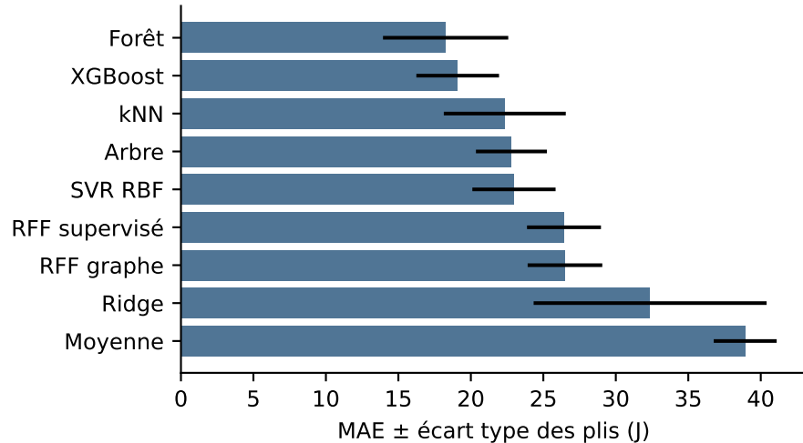
Énergie Charpy
