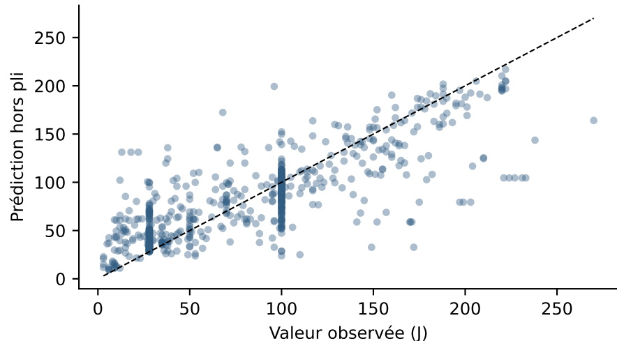
charpy_energy — Forêt
