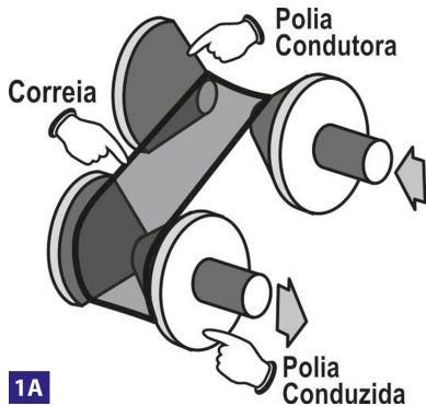
Figura: Conjunto de polias cônicas.
