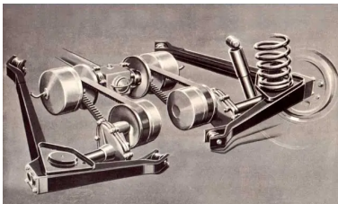
Figura: Sistema DAF Variomatic antigo.
