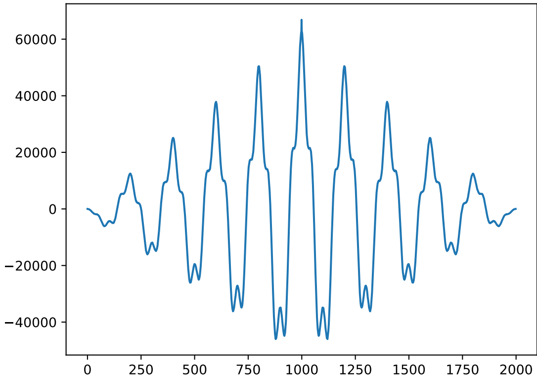
Vectorul de autocorelatie
