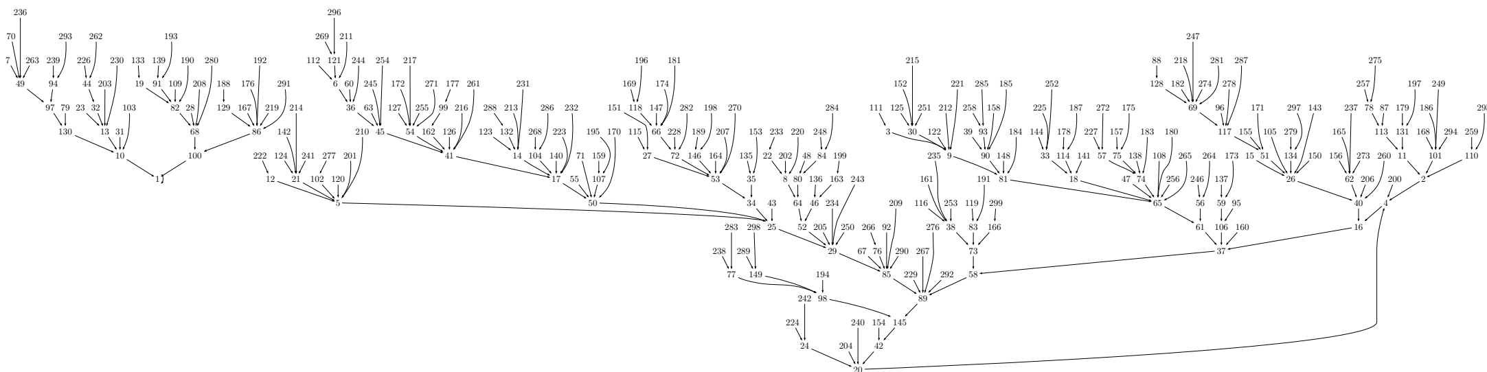
Fig. 1. – Graphe fonctionnel de l’algorithme pour les 300 premiers entiers (on remarque bien qu’il n’existe pas de noeud de degré sortant 0 hormis pour le puits 1)
