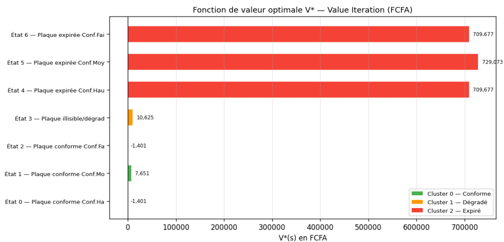
Figure 2.5: Fonction de valeur V^*(s) — Value Iteration ( \gamma = 0.95 ). Les états du cluster 2 (plaques expirées) présentent les valeurs les plus élevées, reflétant le potentiel de recouvrement fiscal DGI.
