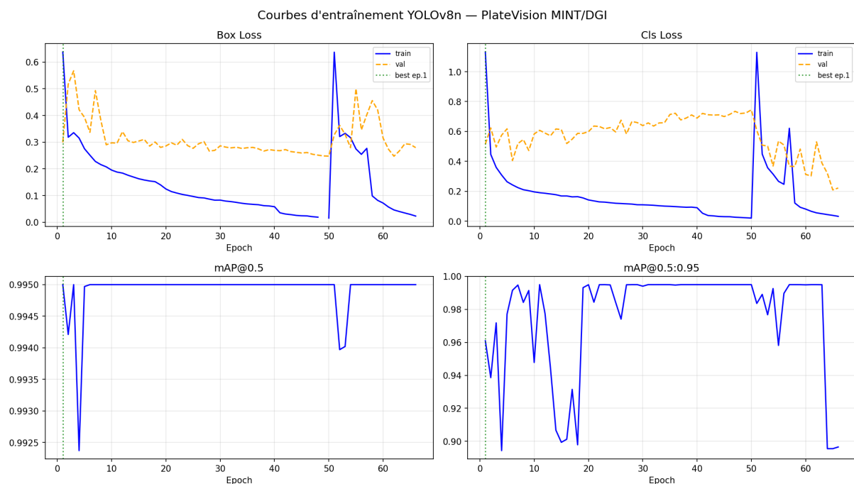
Figure 1.2: Courbes d'entraînement YOLOv8n : pertes box_loss et cls_loss (train/val) et métriques mAP@0.5 / mAP@0.5:0.95 en fonction des epochs. La ligne verte indique l'epoch du meilleur mAP@0.5 ( best.pt ).
