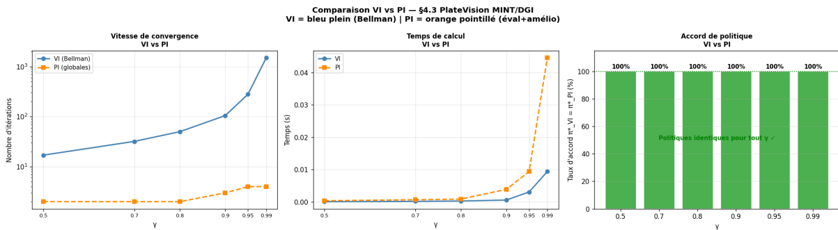
Figure 2.12: Comparaison VI vs PI — vitesse, temps de calcul et accord politique par \gamma
