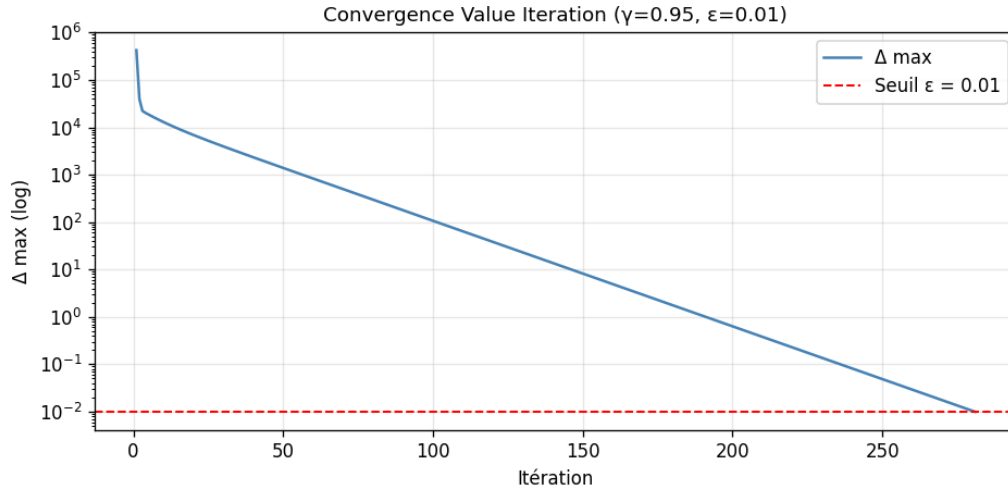
Figure 2.4: Courbe de convergence Value Iteration — variation \Delta V par itération ( \gamma = 0.95 , \varepsilon = 0.01 ). Convergence en 281 itérations.
