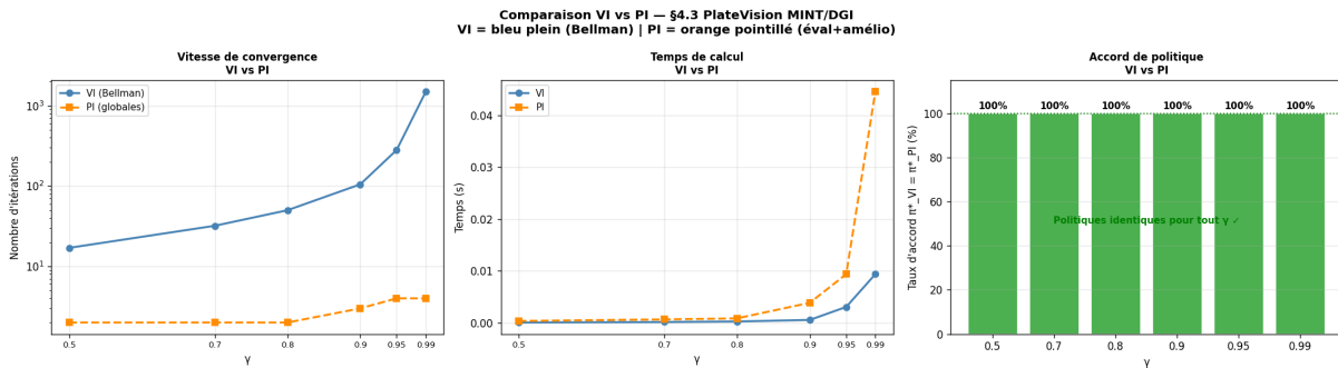
Figure 2.11: Comparaison VI vs PI — vitesse, temps de calcul et accord politique par \gamma
