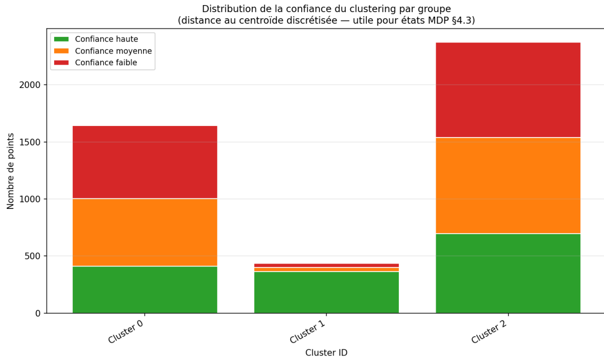
Figure 1.10: Distribution des niveaux de confiance par cluster (confiance = proximité au centroïde K-Means)
