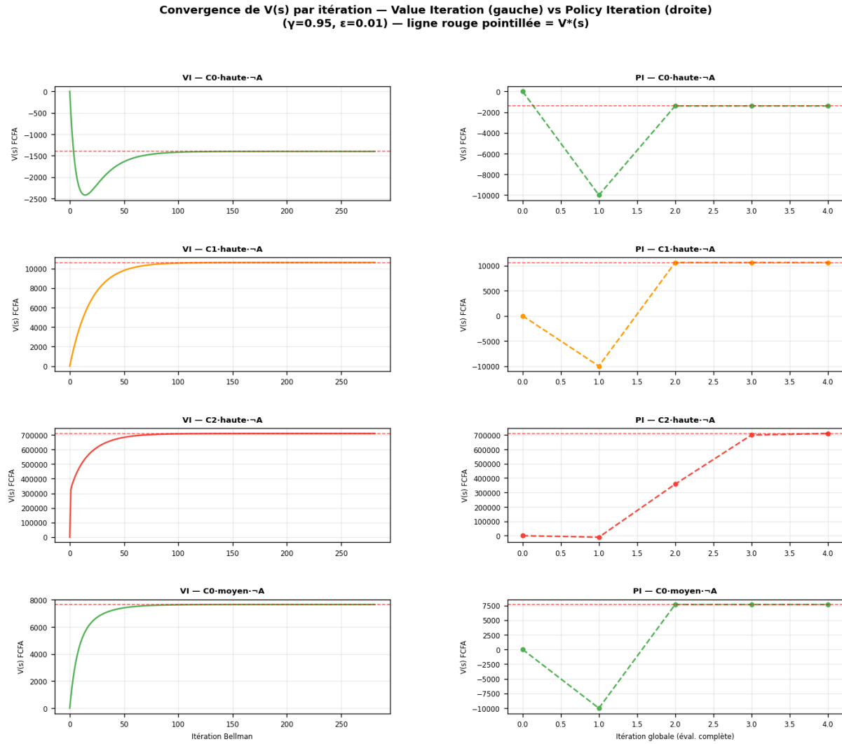
Figure 2.10: Convergence de V(s) par itération — VI (gauche) vs PI (droite)
