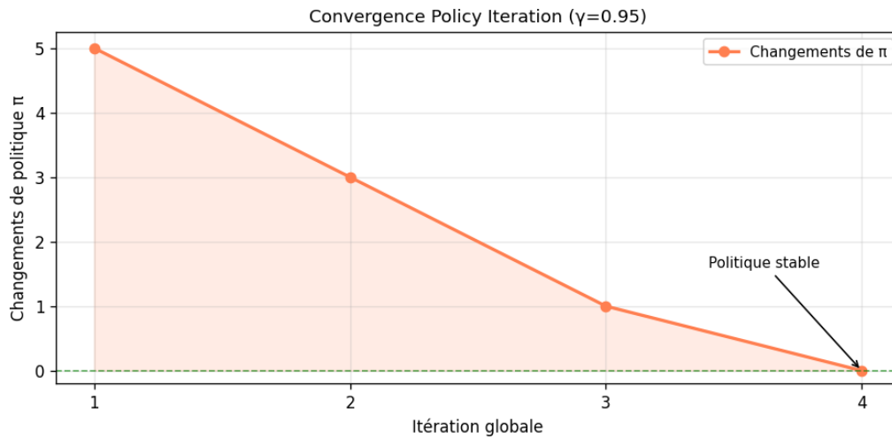
Figure 2.7: Convergence Policy Iteration ( \gamma = 0.95 ) : nombre de changements de politique par itération globale. Stabilisation en 4 itérations (1 735 itérations d'évaluation cumulées).
