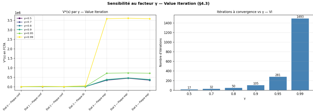
Figure 2.6: Sensibilité de Value Iteration au facteur \gamma : nombre d'itérations jusqu'à convergence pour \gamma \in \{0.50, 0.70, 0.80, 0.90, 0.95, 0.99\} . La politique \pi^* reste stable pour tout \gamma \geq 0.70 .
