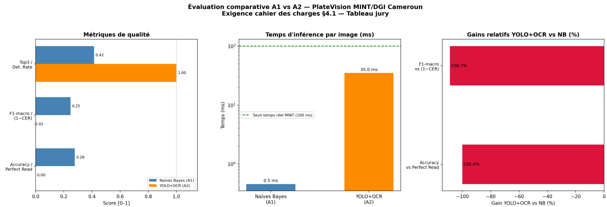
Figure 1.3: Évaluation comparative Naïves Bayes (A1) vs YOLO+OCR (A2). Panneau gauche : métriques de qualité (accuracy/perfect read rate, F1/1-CER, top3/detection rate). Panneau centre : temps d'inférence par image (ms) avec seuil temps réel MINT à 100 ms. Panneau droit : gains relatifs YOLO+OCR vs NB (%).
