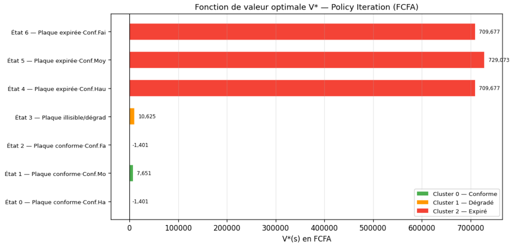
Figure 2.8: Fonction de valeur V^*(s) — Policy Iteration ( \gamma = 0.95 ). Identique à celle obtenue par VI : valeurs élevées pour les états d’infractions fiscales (cluster 2, plaques expirées).
