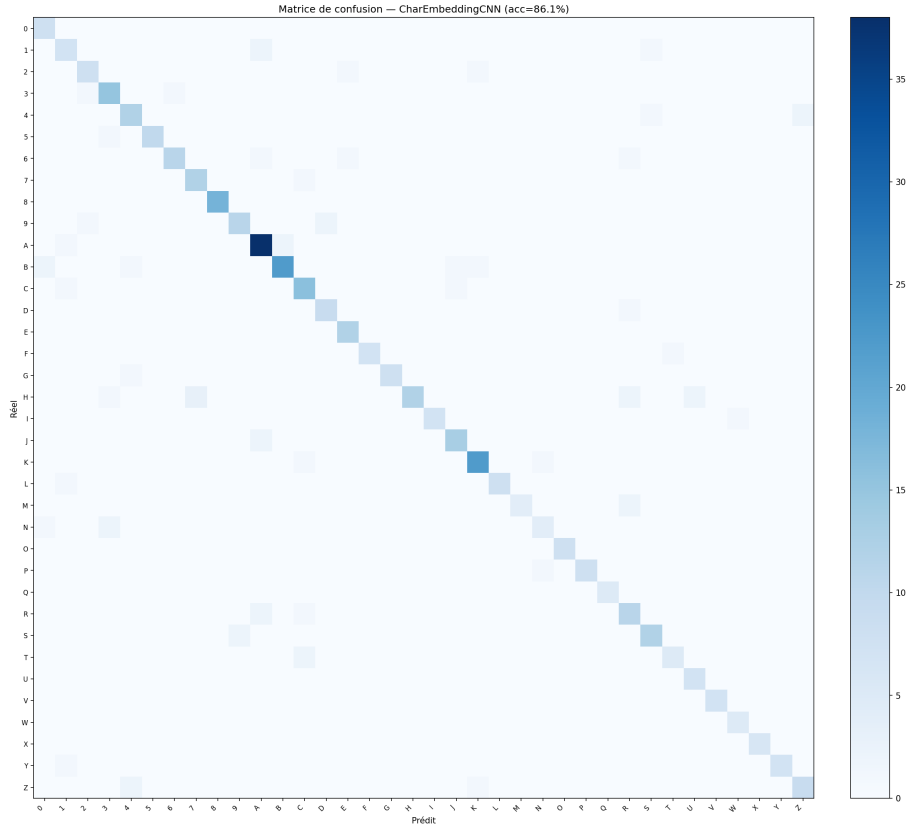
Figure 1.4: Matrice de confusion du CNN CharEmbeddingCNN sur le jeu de test (36 classes alphanumériques) — exercice pédagogique Module A1/B0, n'alimente plus le clustering
