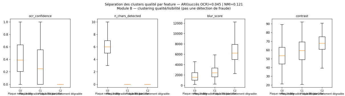
Figure 1.11: Séparation des 4 features de qualité par cluster K-Means (ARI = 0,045, NMI = 0,121 vs. succès OCR) — §4.2 : le clustering sépare-t-il bien le signal de lisibilité ?
