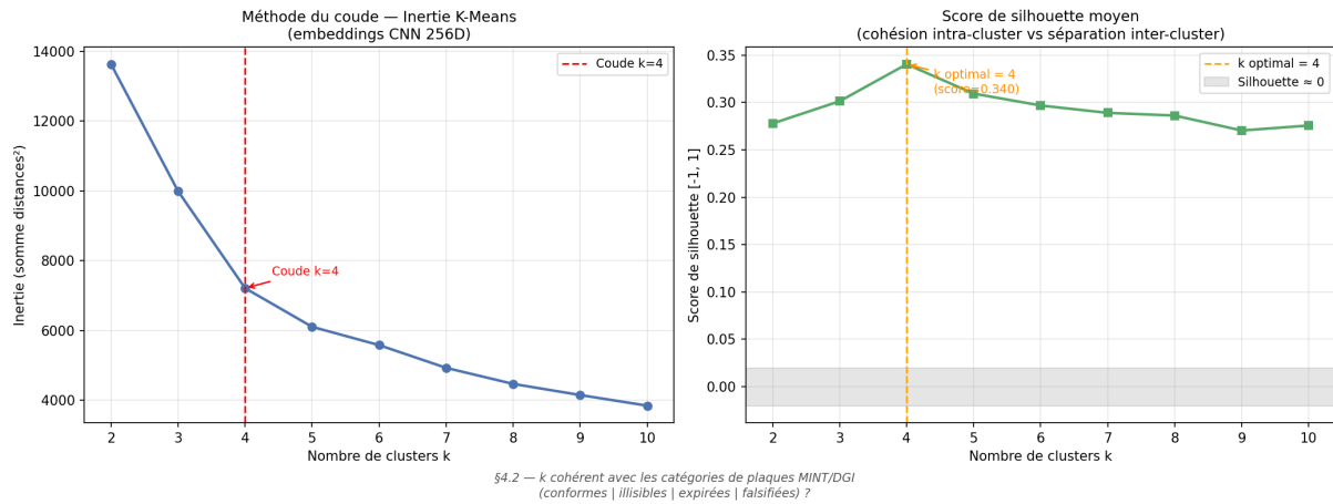
Figure 1.5: Méthode du coude et score de silhouette — détermination de k optimal (Module B PlateVision)
