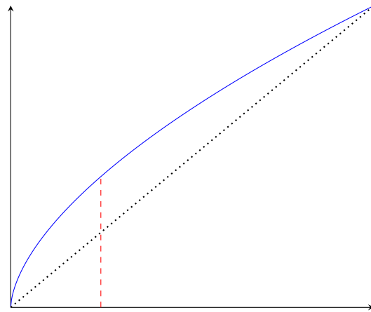
(d) q^\beta - (2, 2, 1)
