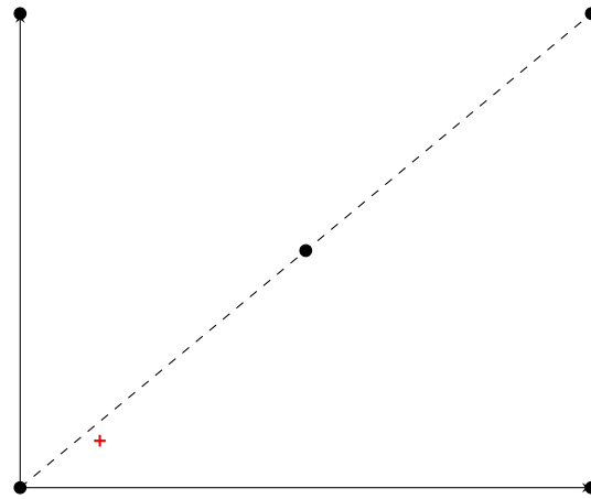
(d) RecLMTD - (2, 2, 1)
